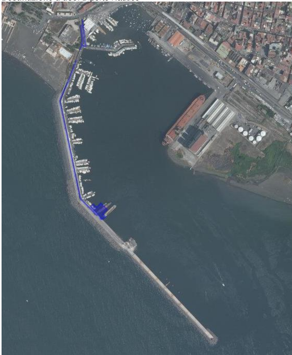
- Planimetria di inquadramento Porto di Torre Annunziata
