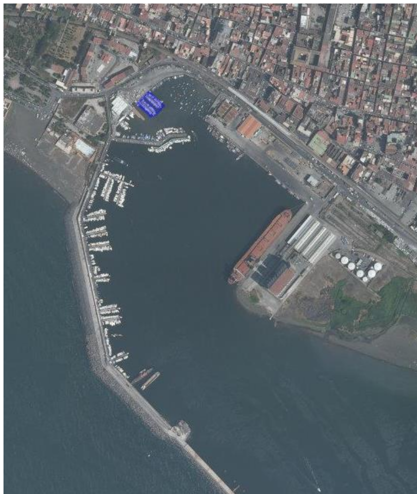
-Planimetria di inquadramento Porto di Torre Annunziata
