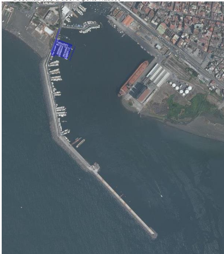
- Planimetria di inquadramento Porto di Torre Annunziata
