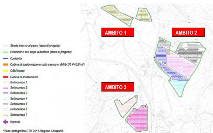
Fig. 7 – Suddivisione del layout di progetto in ambiti e sottocampi (Fonte: PVFRAG-P17.02-00 - LAYOUT DI PROGETTO CON SOTTOCAMPI)
