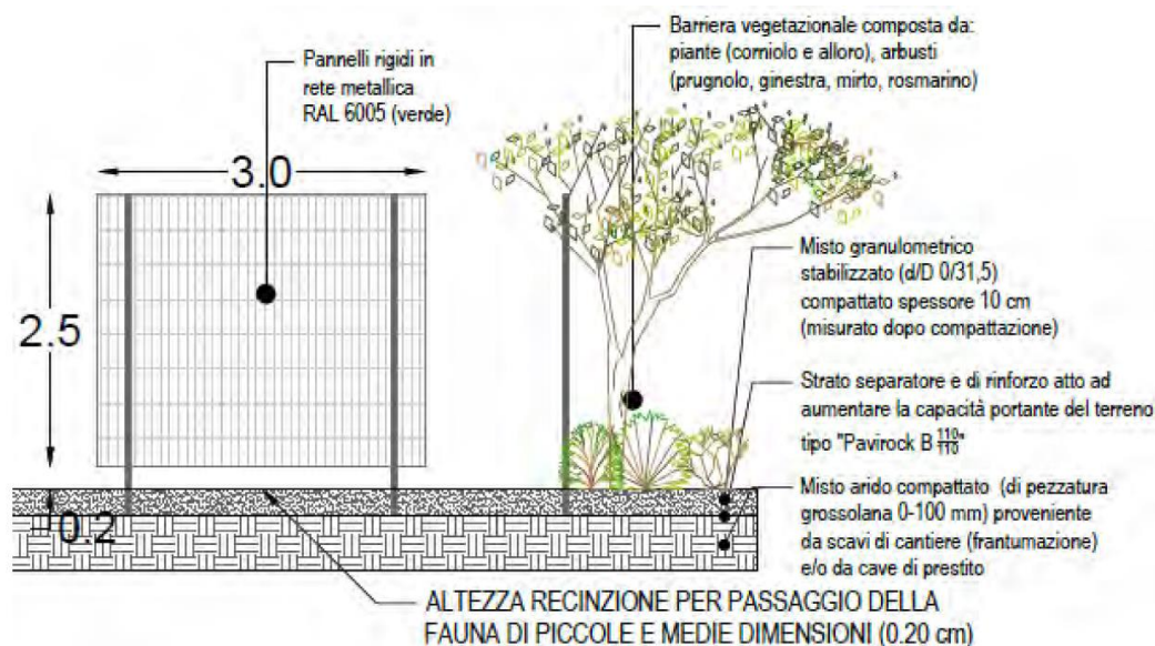
Figura 6 – schema recinzione
