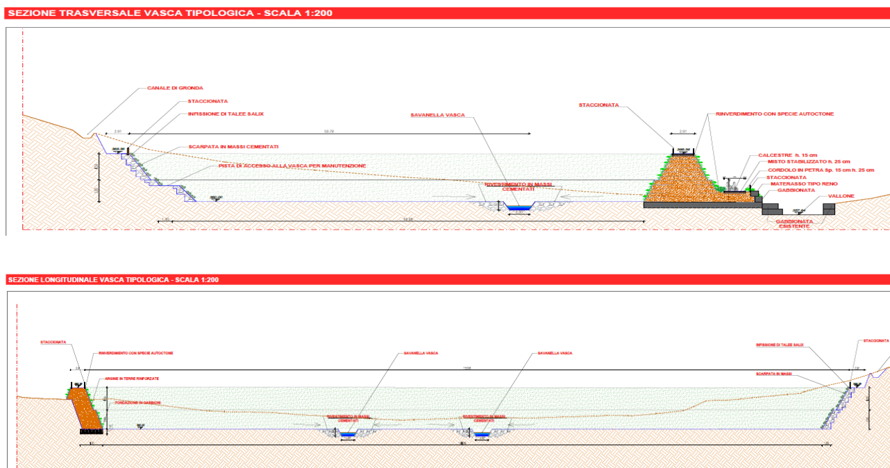
Figura 1.3.2 – Sezioni tipo vasca di laminazione (trasversale e longitudinale)
