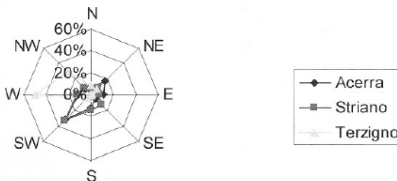
Figura 6- Frequenze dei venti registrate ad Acerra Striano e Terzigno nel periodo 1999-2002 (Fonte: ISTAT)
