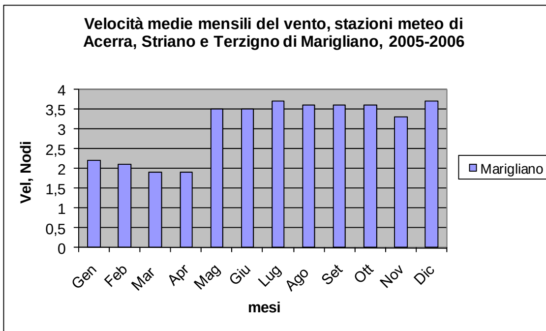
Figura 9- velocità media del vento Marigliano (Fonte : ISTAT)
