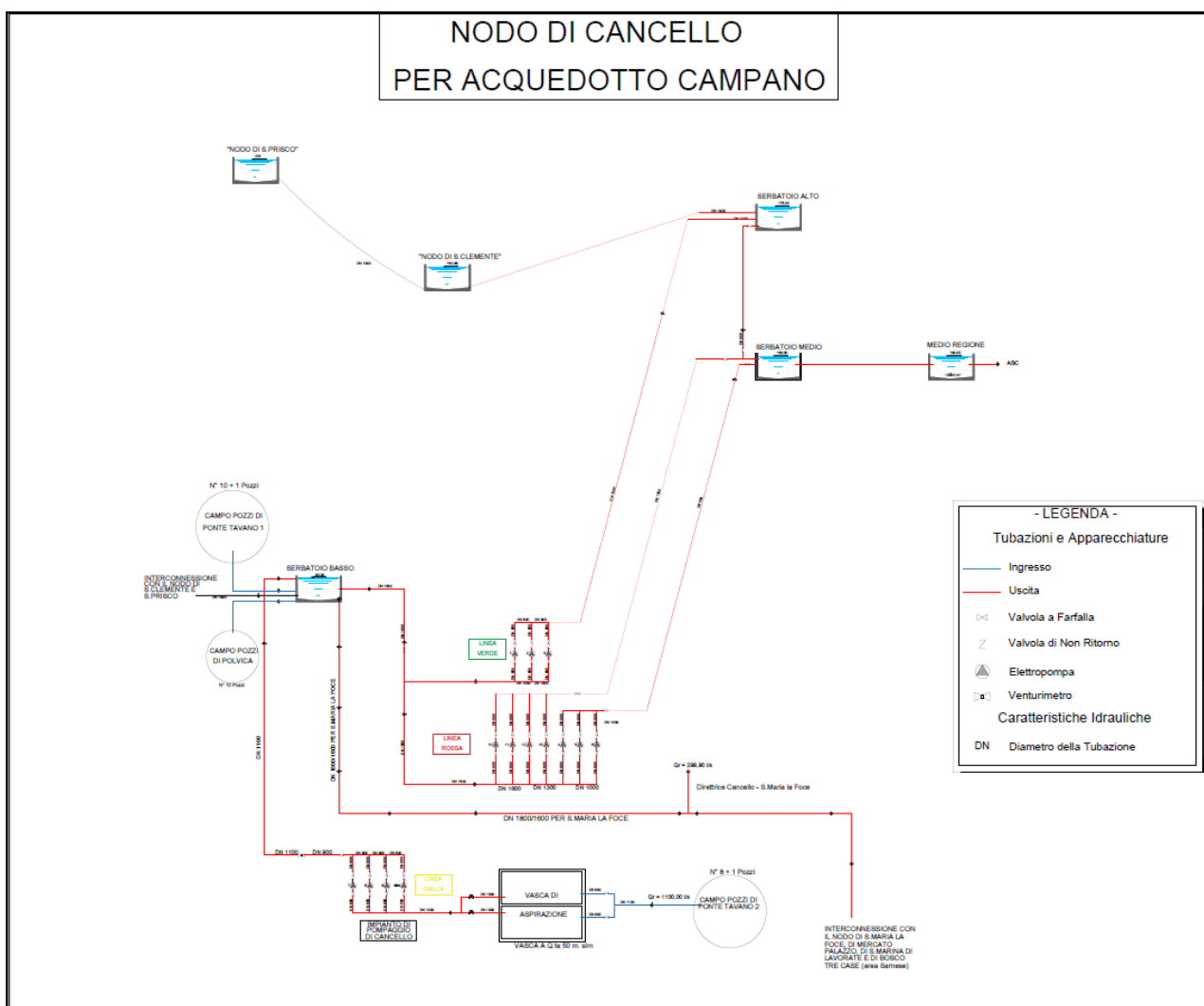
Nodo di Cancellone - Schema generale 1
