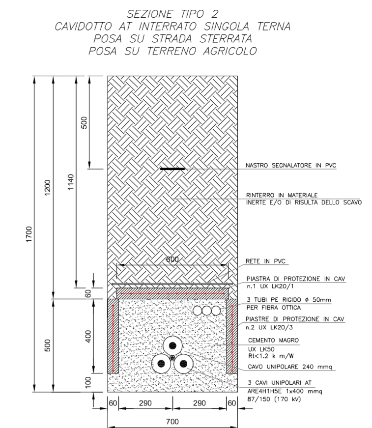
PARTICOLARE A: Sezioni cavidotto AT - scala 1:20
