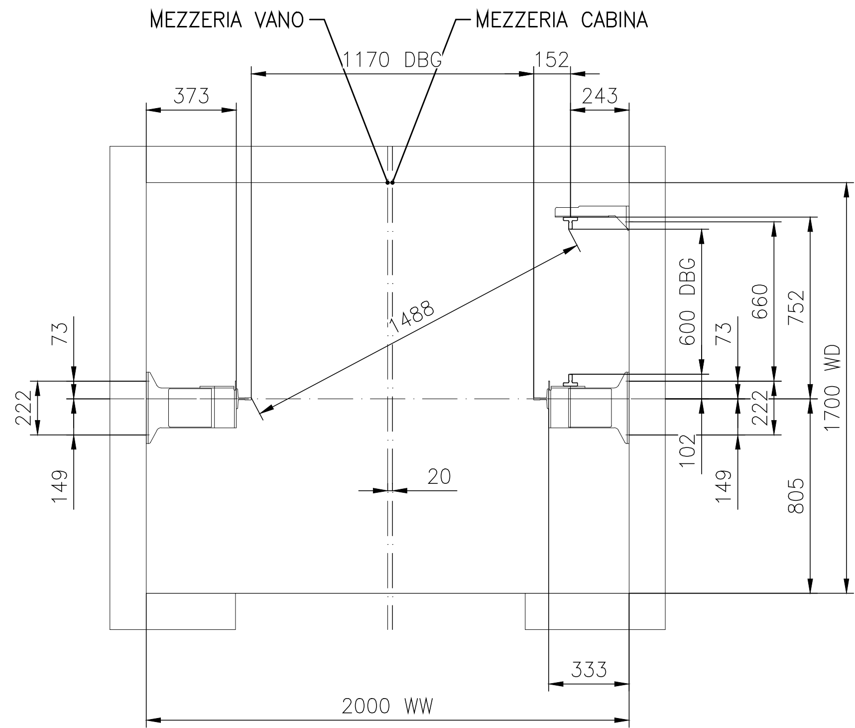
A LATO GUIDE Scala 1:30
