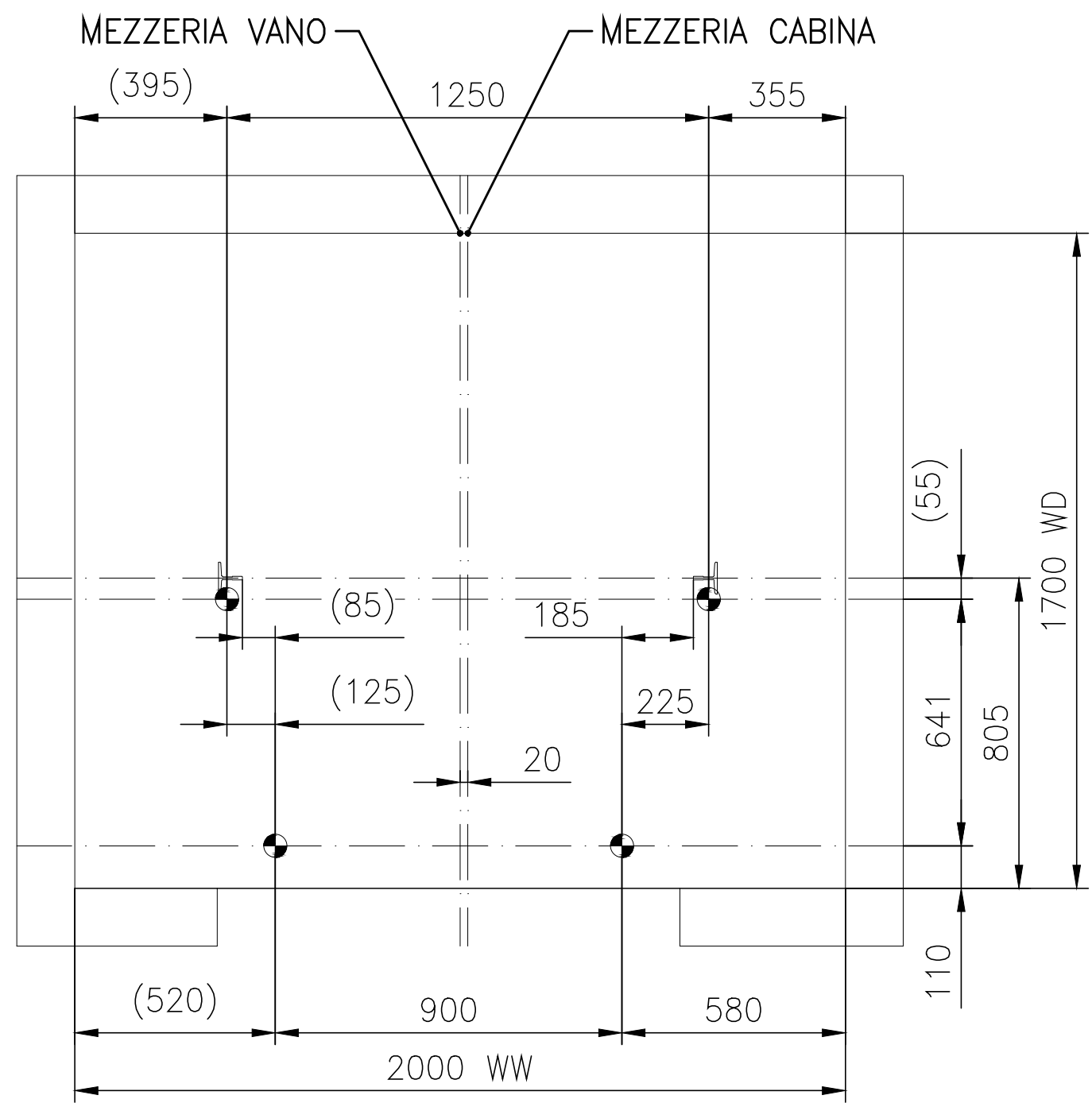
A LATO FILO PIOMBO Scala 1:30
