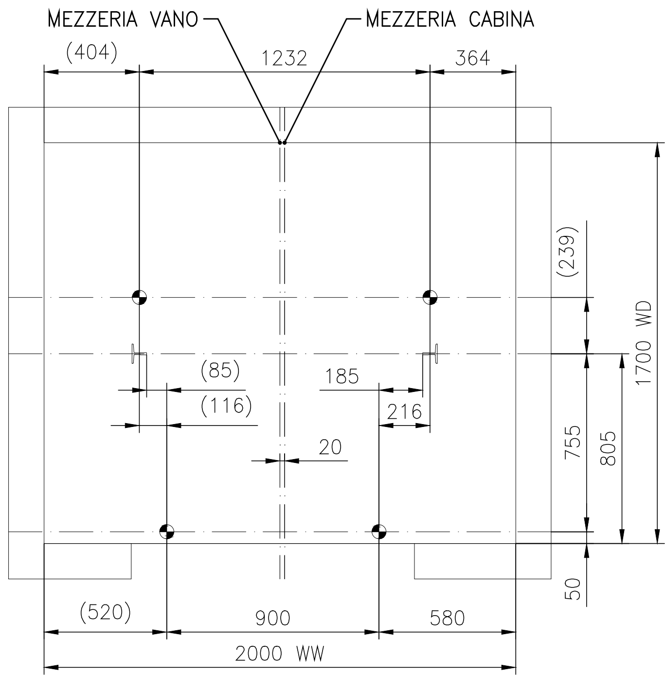
A LATO LASER PIOMBO Scala 1:30
