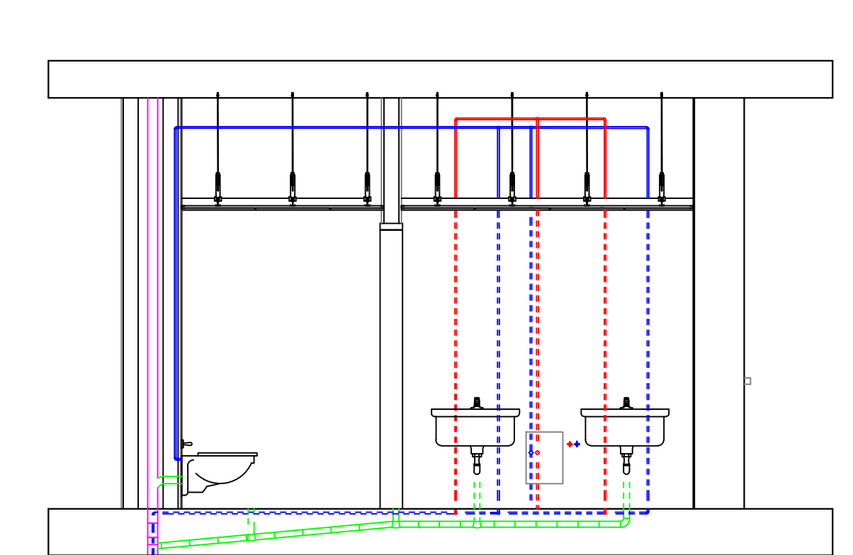
SEZIONE B-B SCHEMA FUNZIONALE
