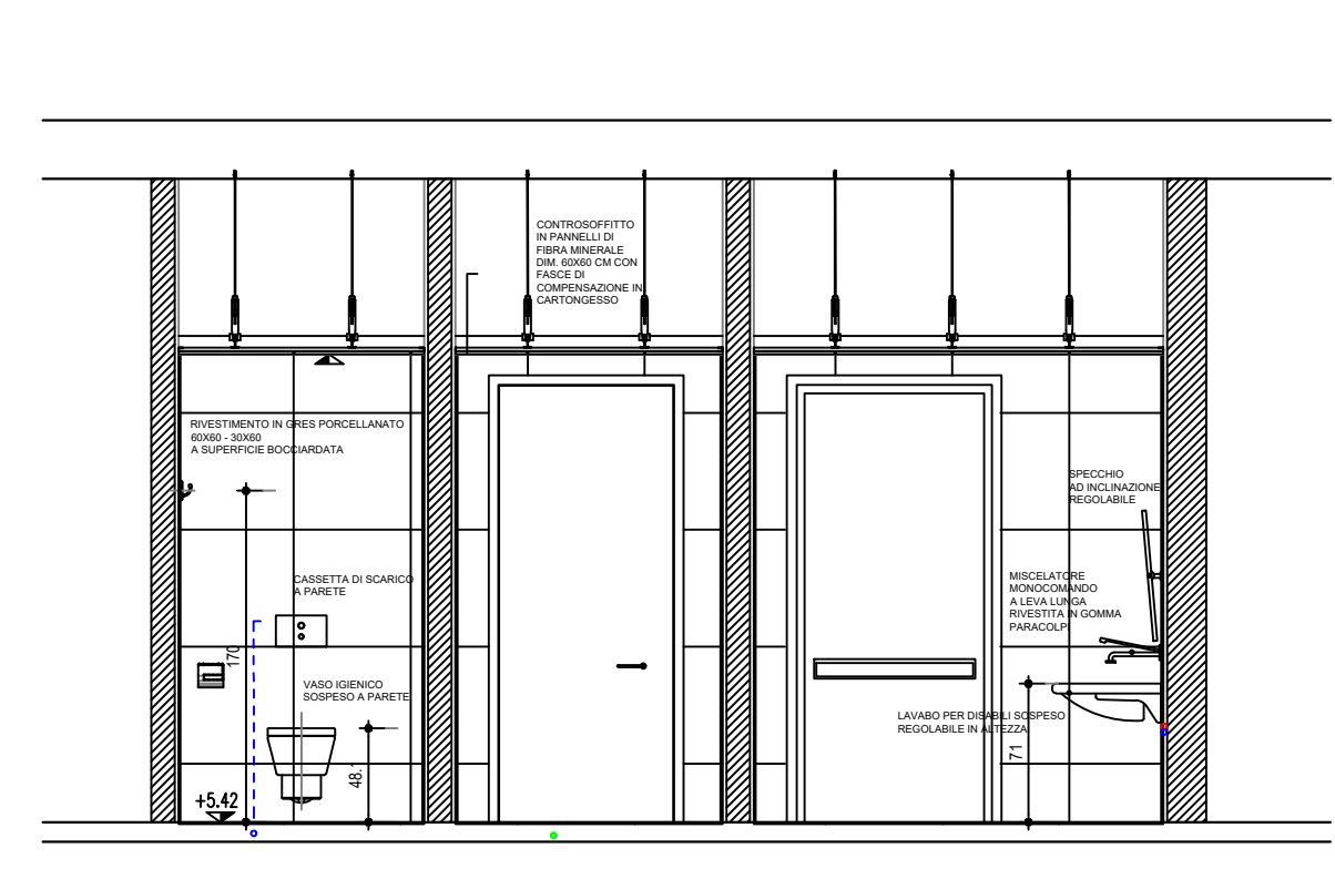
SEZIONE A-A
