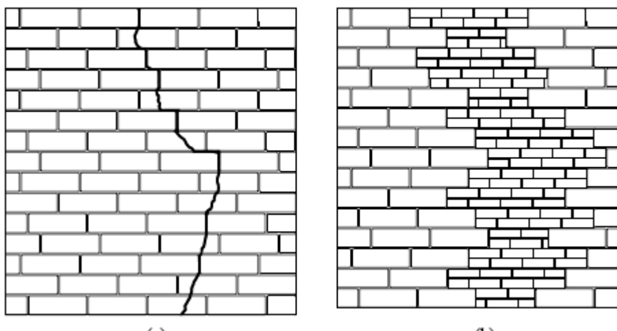
. Paramento murario oggetto di intervento di scuci e cucì: a) prima dell'intervento; b) dopo l'intervento
