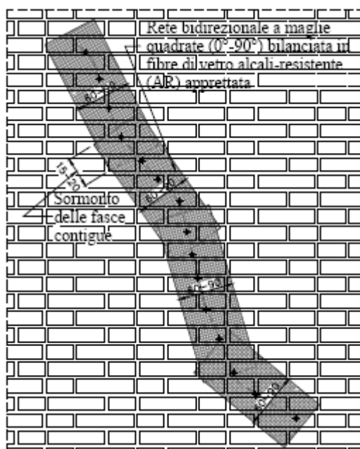
Applicazione di rete di rinforzo: vista prospettica
