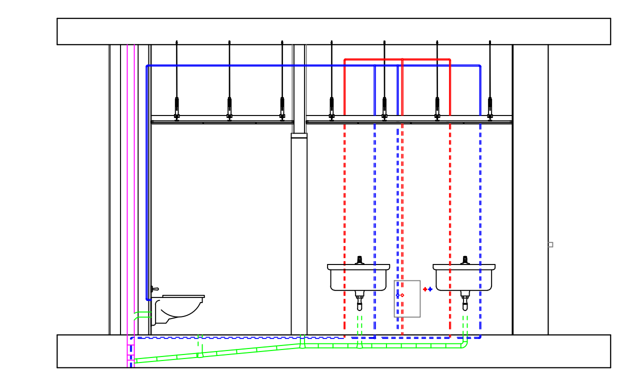
SEZIONE B-B SCHEMA FUNZIONALE
