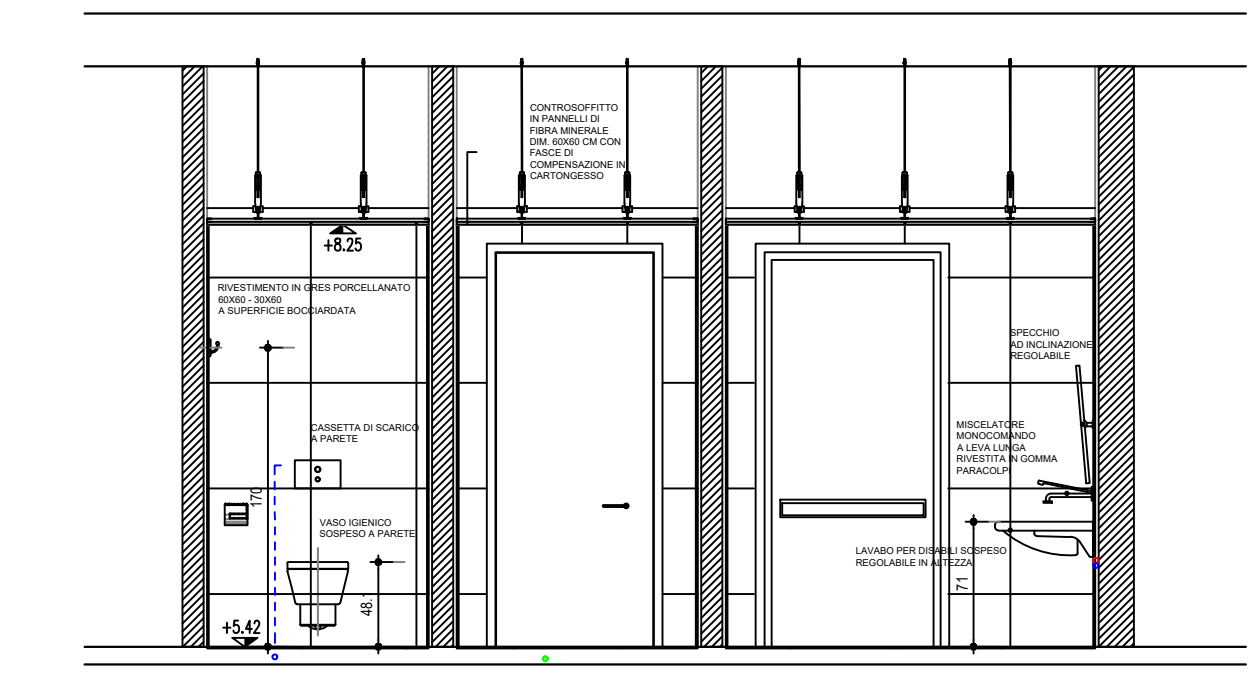
SEZIONE A-A
