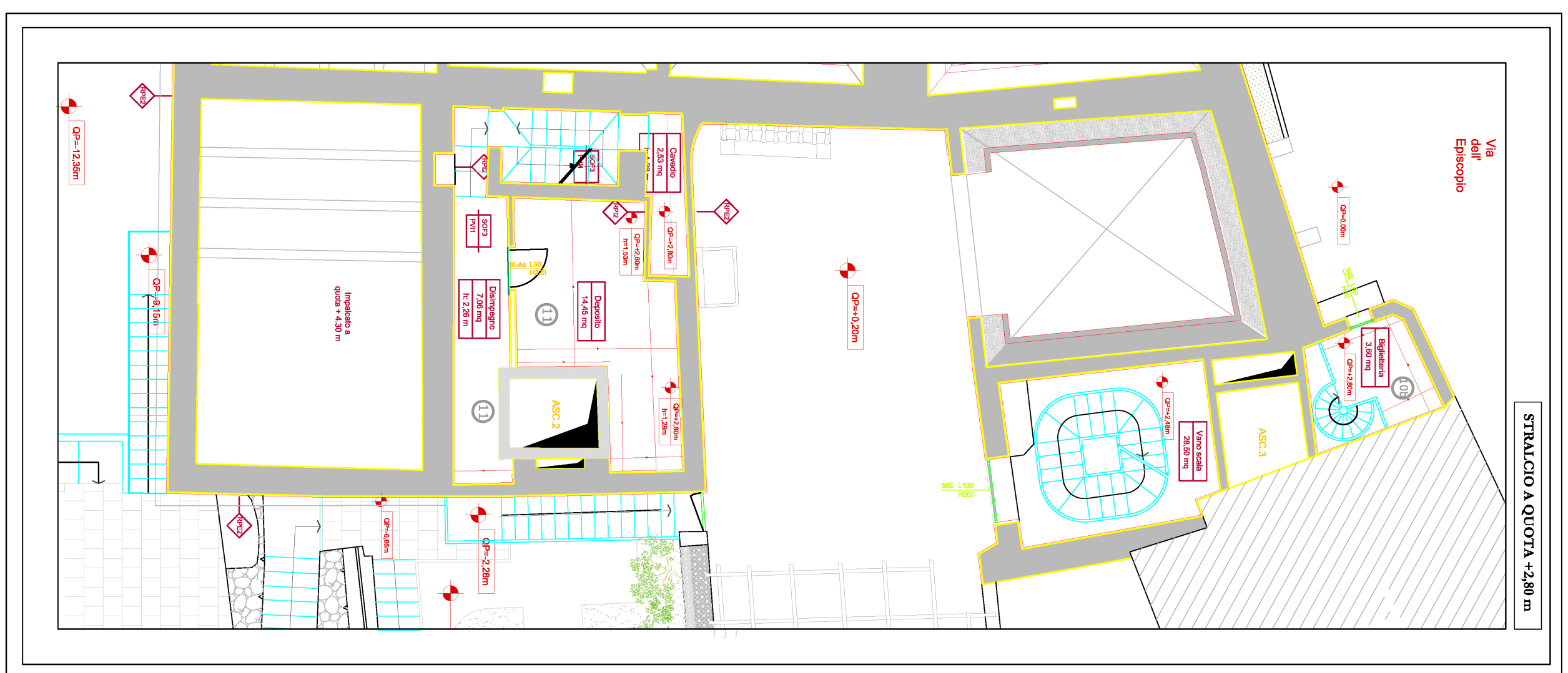
PROGETTO ESECUTIVO Stralcio Elaborato N°: 67 PARE.49 Pianta a quota +5,85 / +2,80 Stralcio Pianta a quota +2,70 scala di rappresentazione: 1:100
