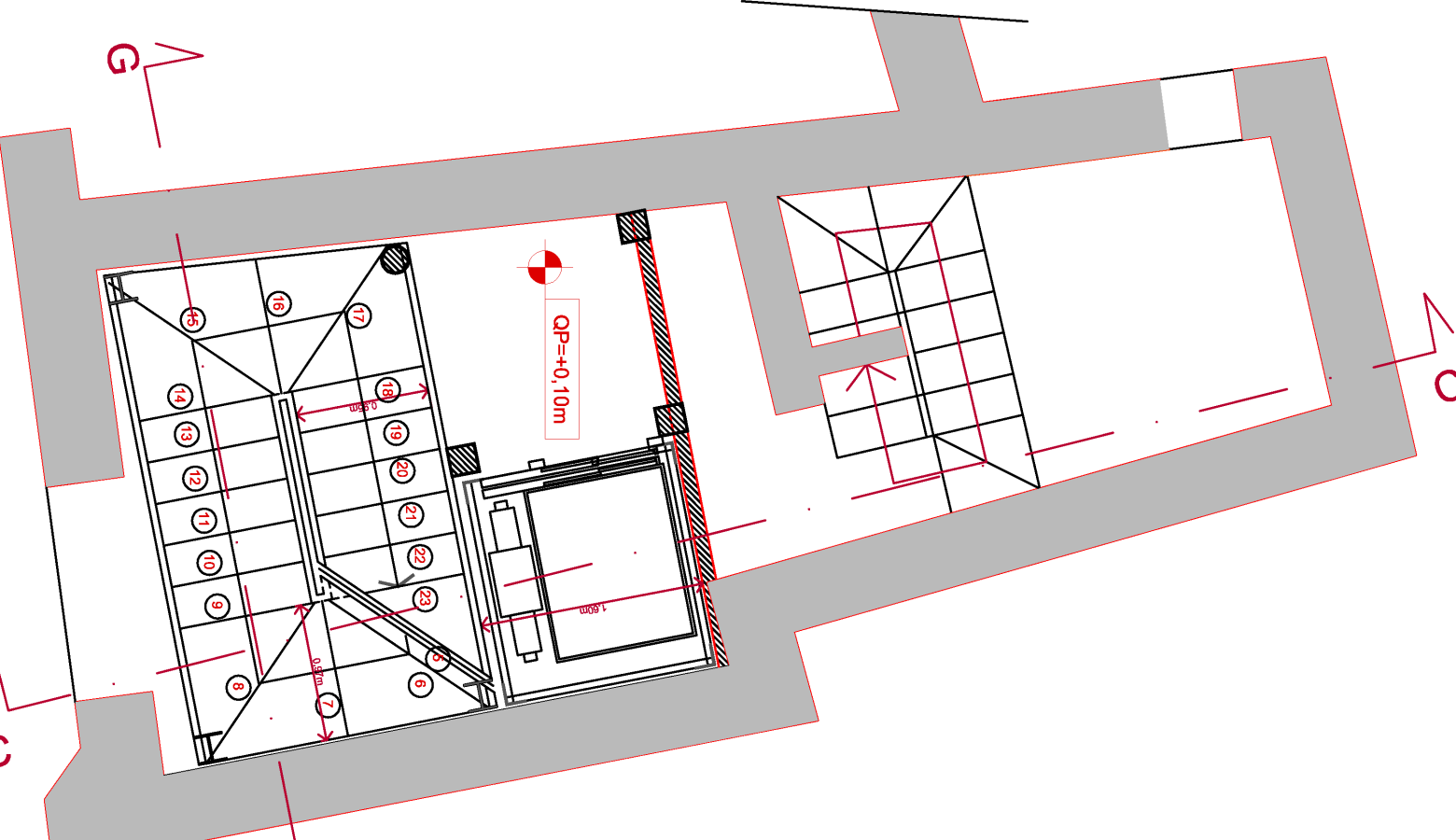
PROGETTO DI VARIANTE Stralcio pianta a quota +2,80 scala di rappresentazione: 1:50
