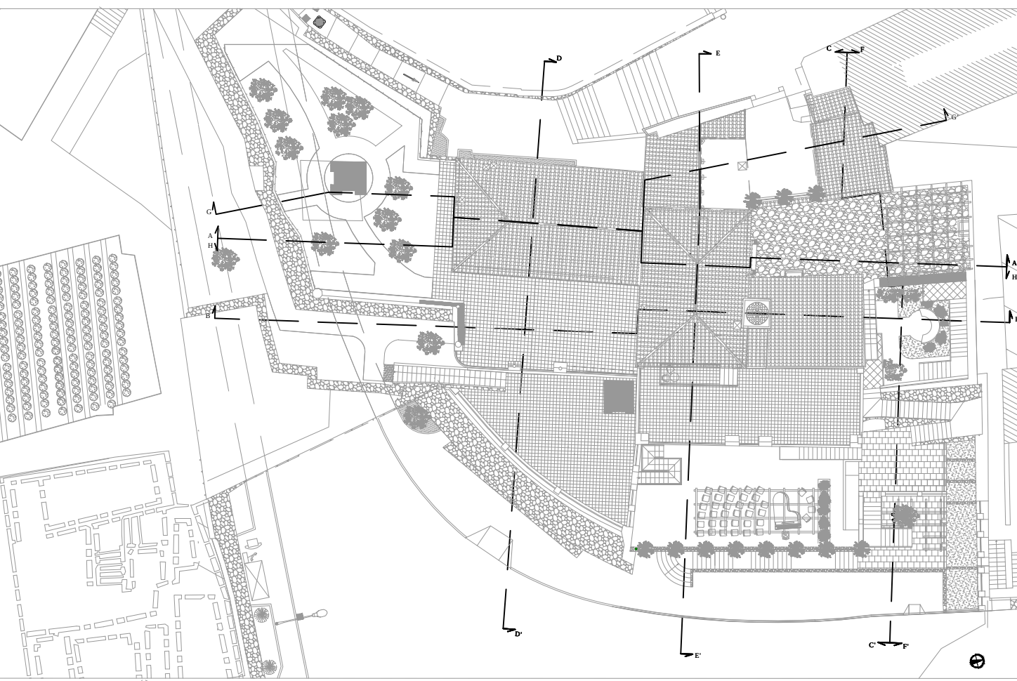
PIANTA DELLE COPERTURE
