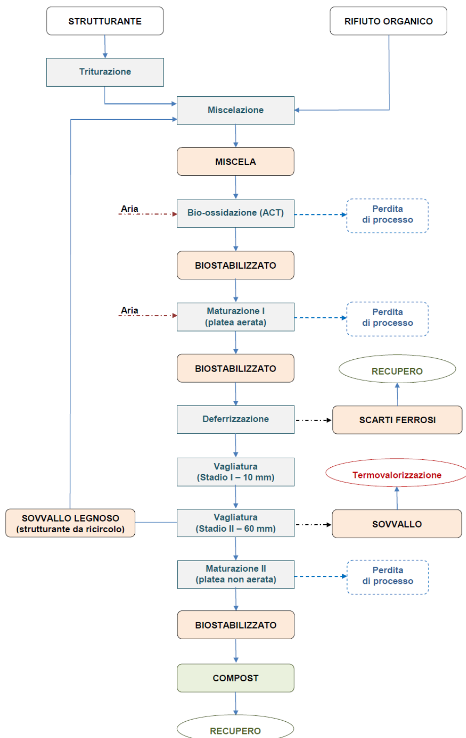
Figura 3 – schema di flusso impianto
