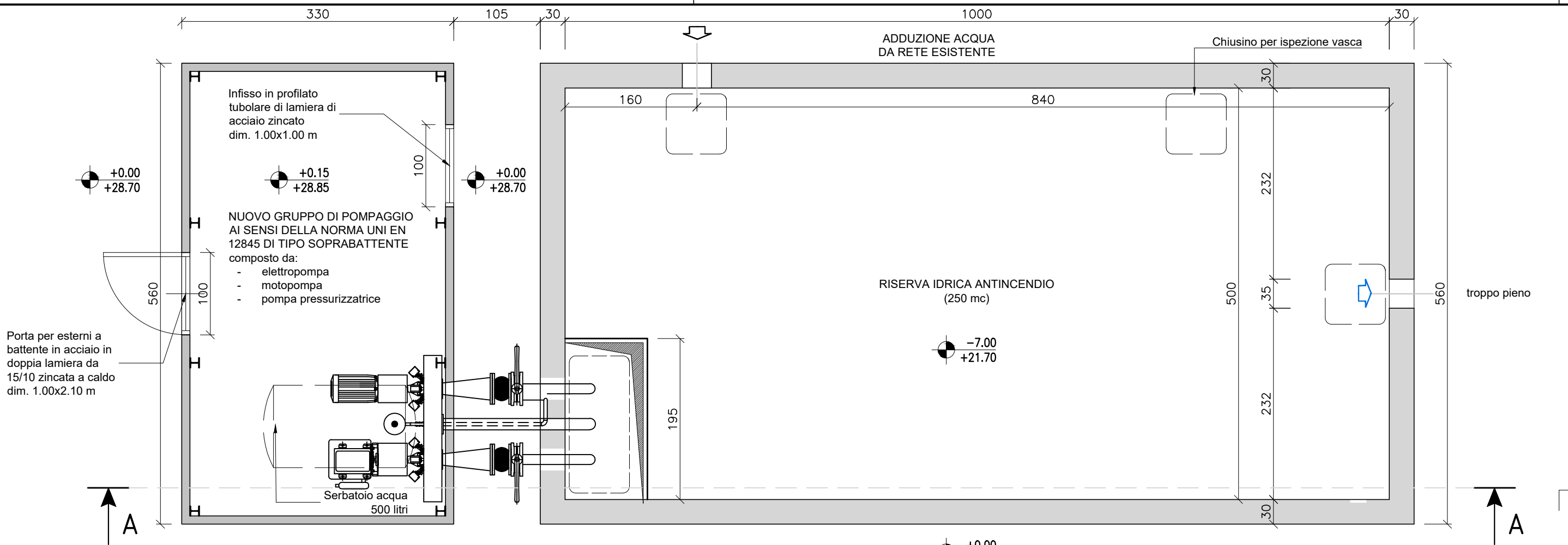
PIANTA SCALA 1:50
