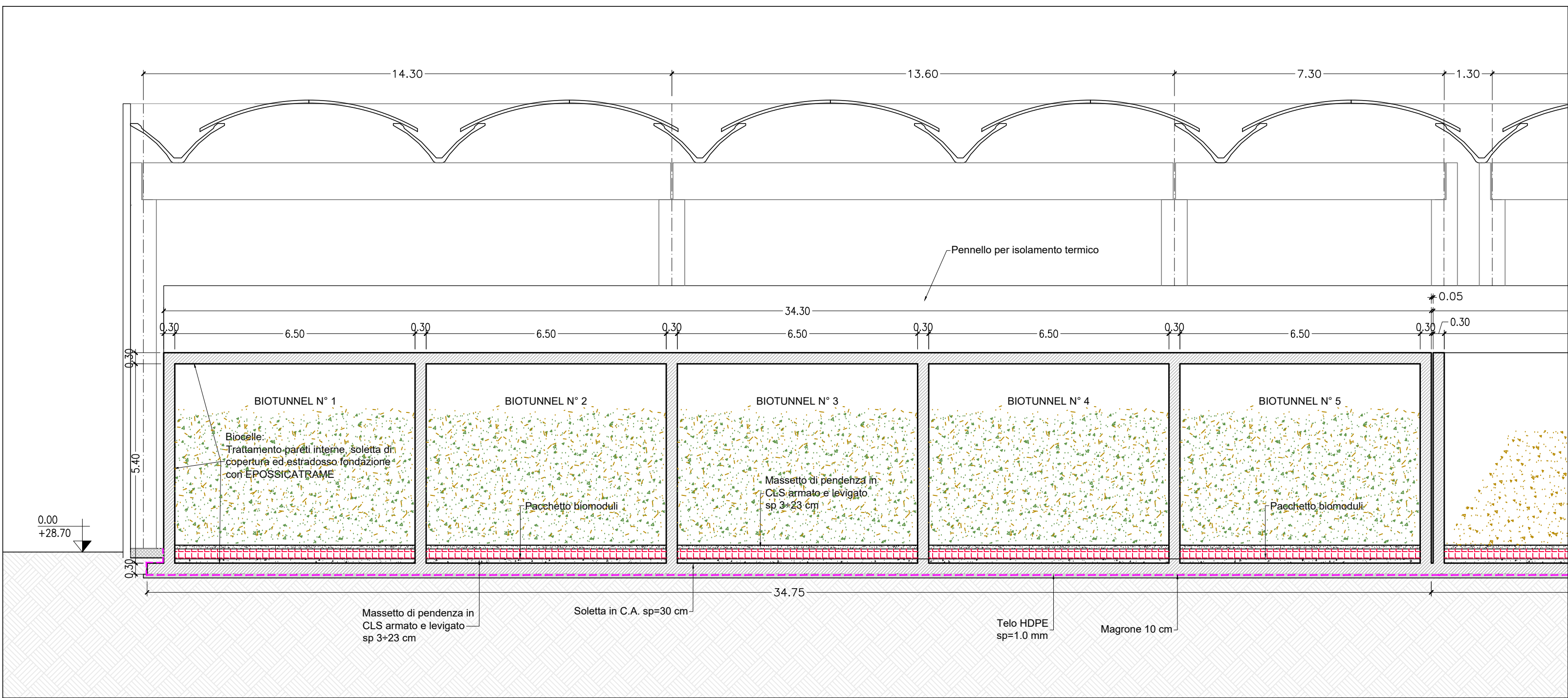
SEZIONE A-A BIOCELLE SCALA 1:100
