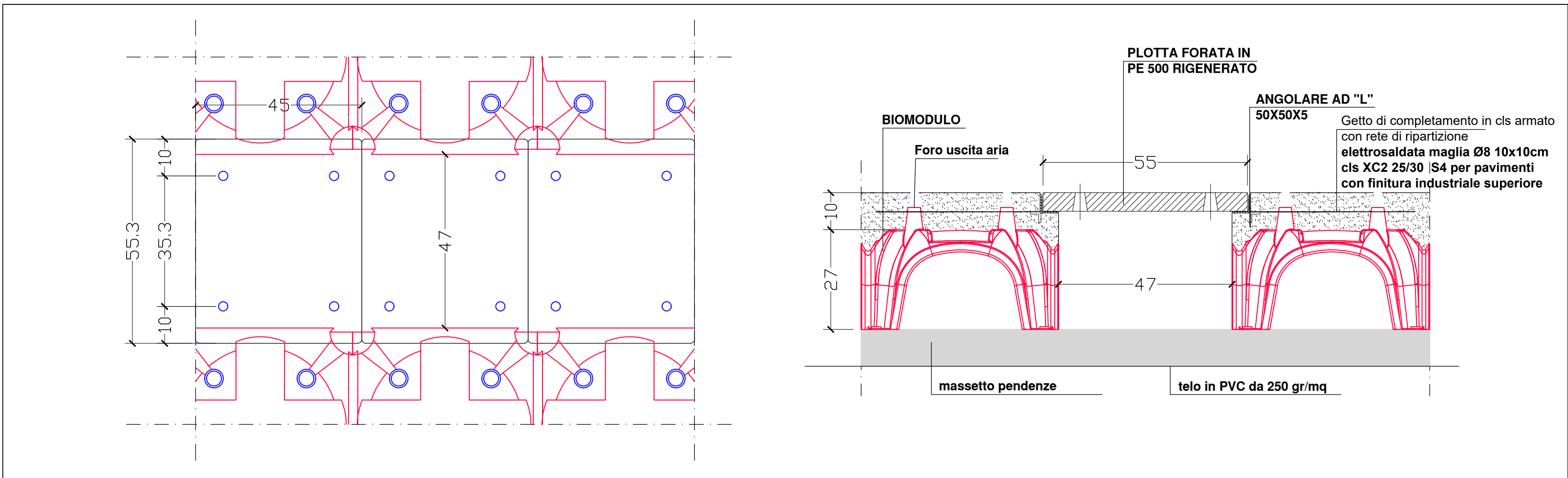
PARTICOLARE TIPO PLOTTA E BIOMODULO TIPO GEOPLAST SCALA 1:10
