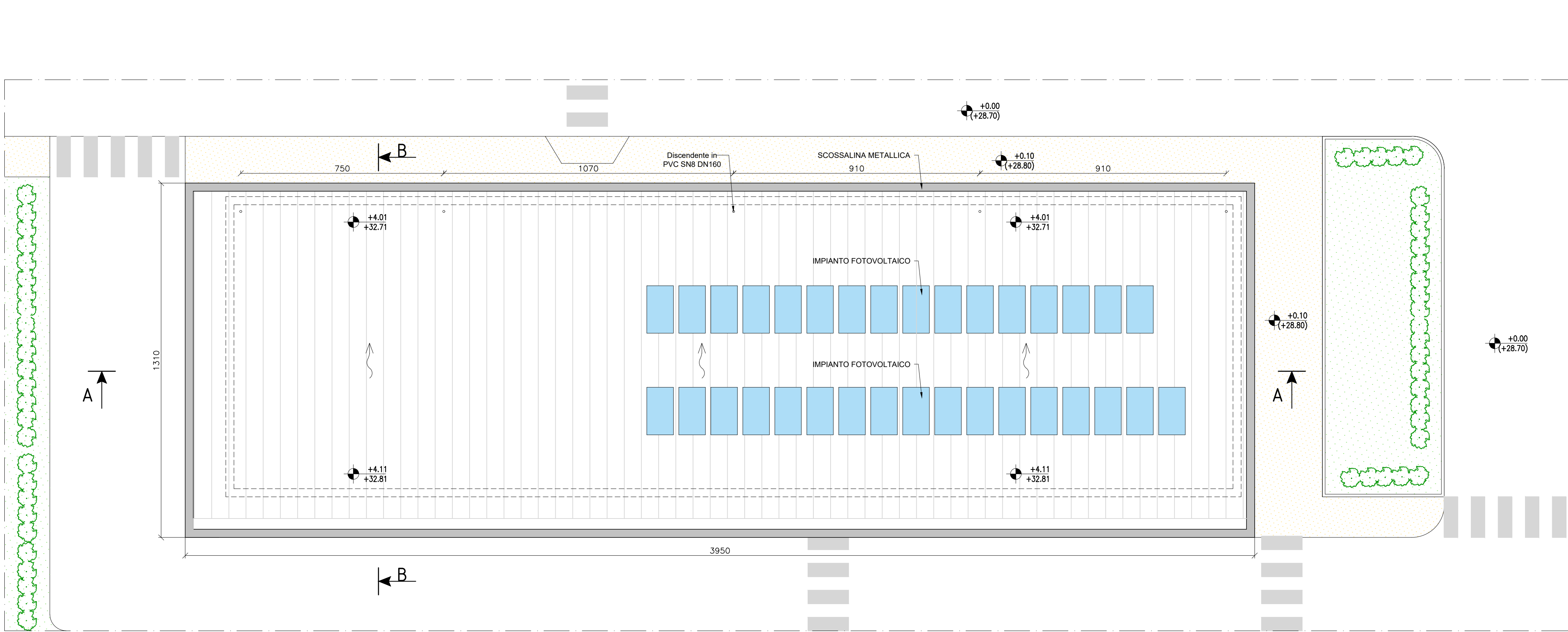
PIANTA COPERTURA SCALA 1:100
