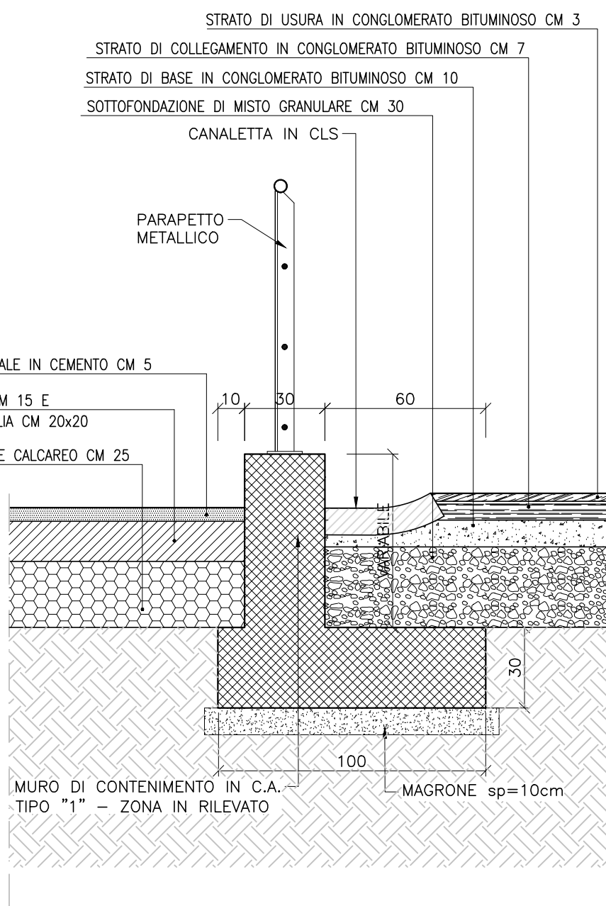
PARTICOLARE MURO "M1" SCALA 1:20
