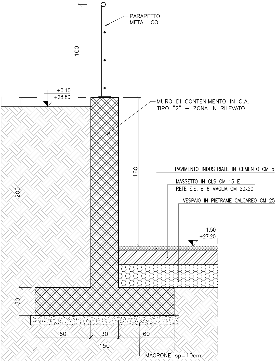
PARTICOLARE MURO "M2" SCALA 1:20
