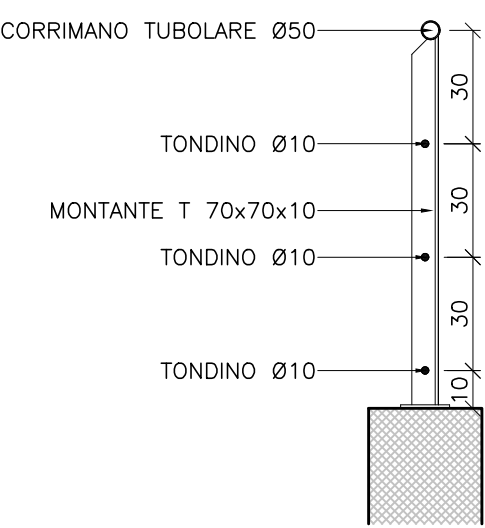
PARTICOLARE MURO "M1" SCALA 1:20
