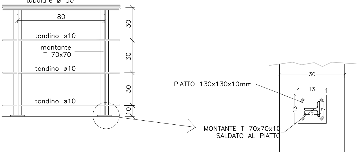
PARTICOLARE PARAPETTO SCALA 1:20
