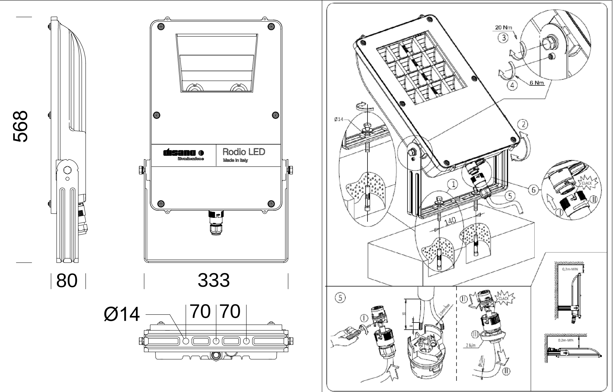
PARTICOLARE INSTALLATIVO - RODIO 1898
