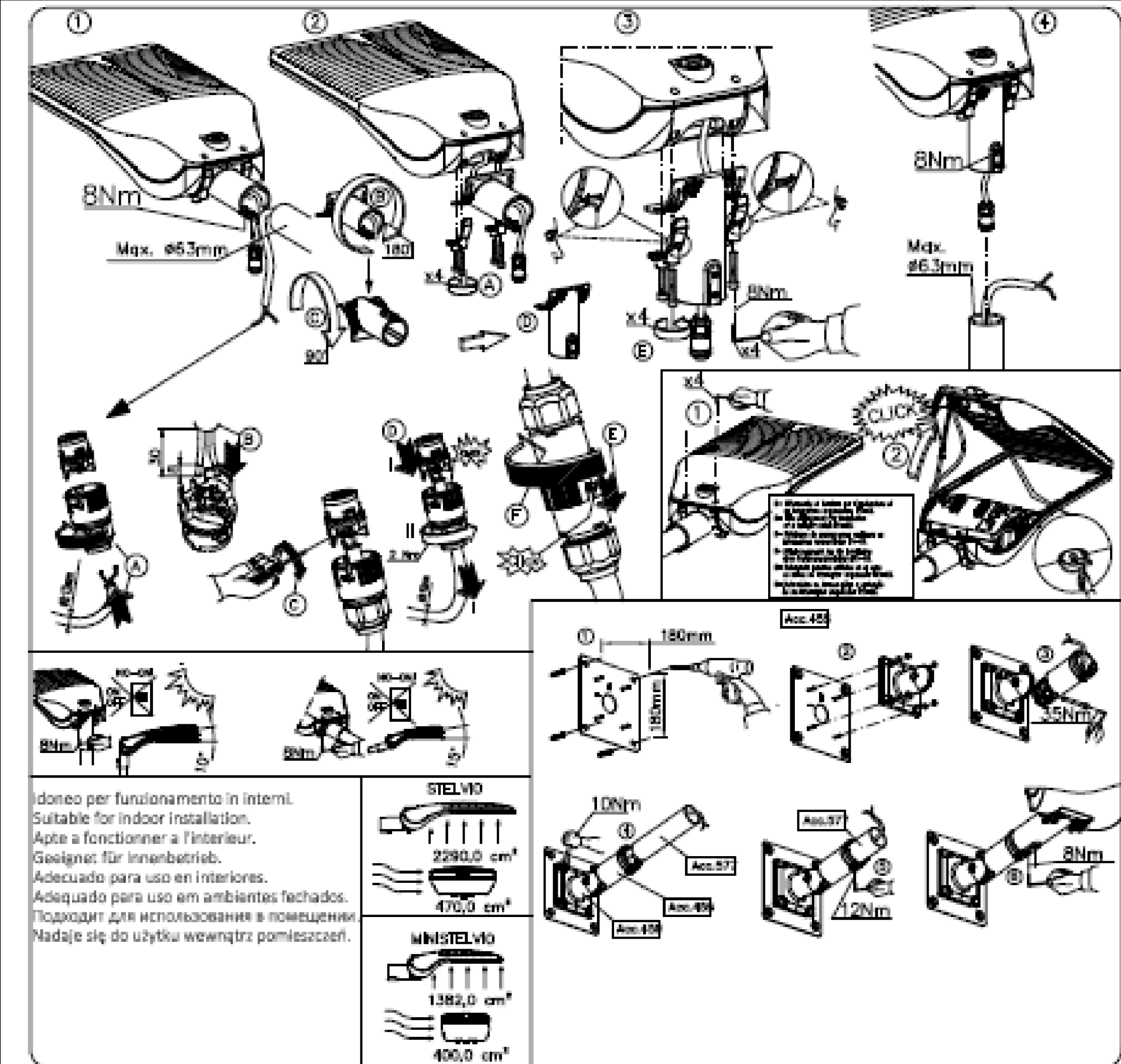
PARTICOLARE INSTALLATIVO - DISANO 3376
