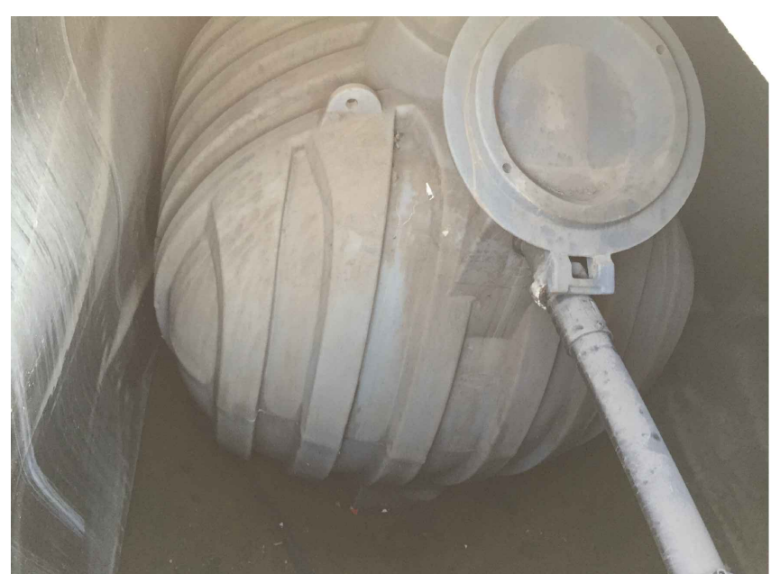
FOTO 5 - INTERNO VASCHE DI RACCOLTA PERCOLATO CON SERBATOI
