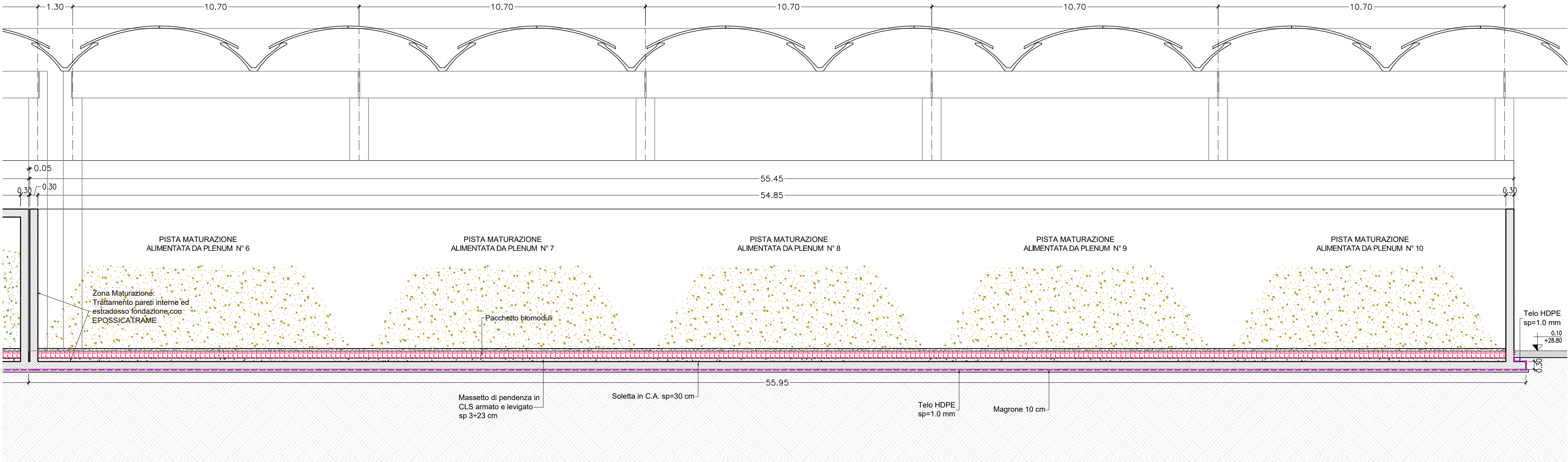
SEZIONE A - A MATURAZIONE PRIMARIA SCALA 1:100
