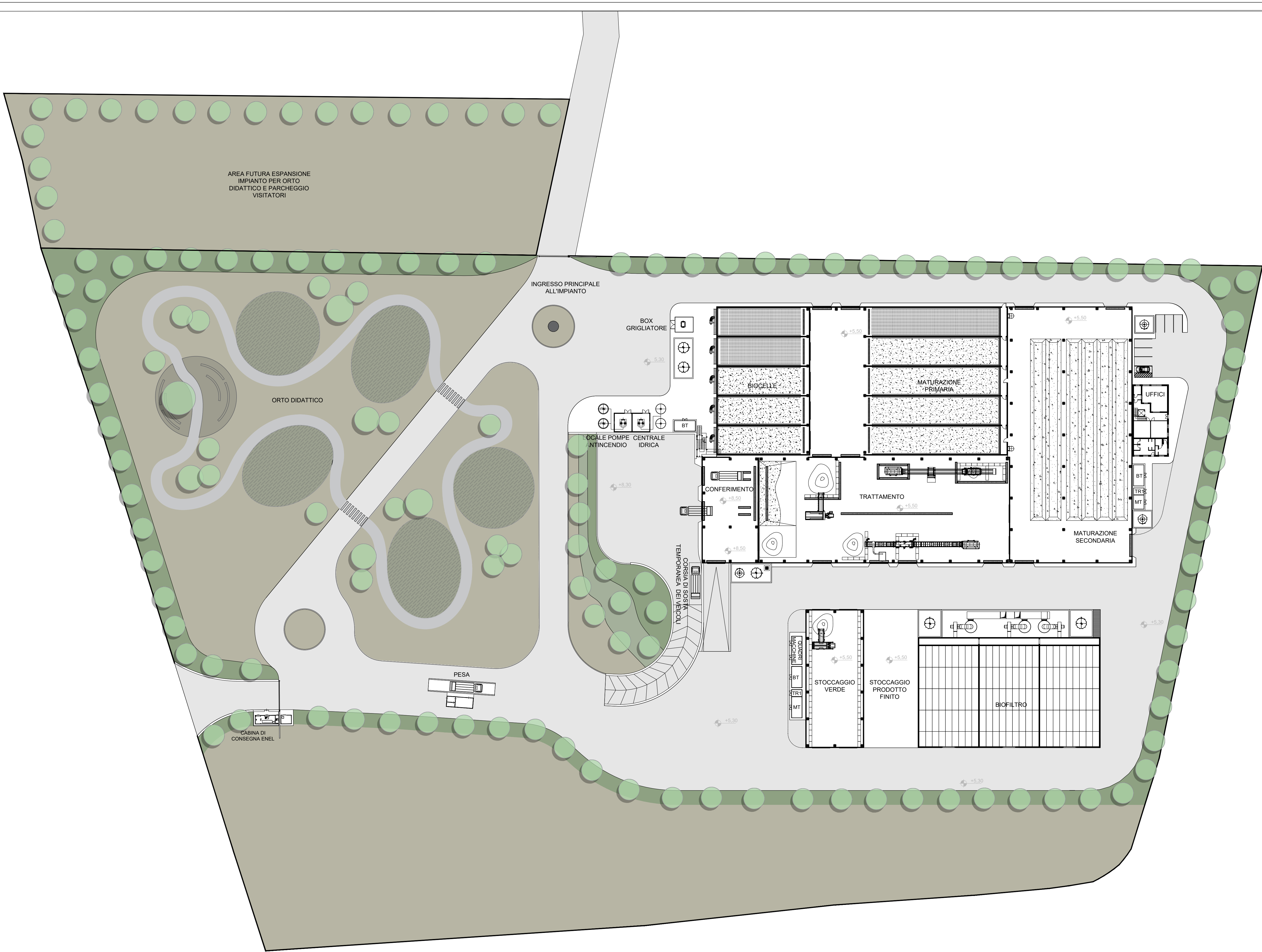
PLANIMETRIA GENERALE - STATO DI PROGETTO
