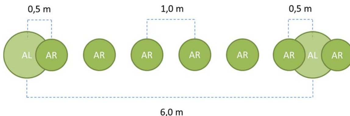
FIGURA 8-42 – SCHEMA DI IMPIANTO DELLA SIEPE
