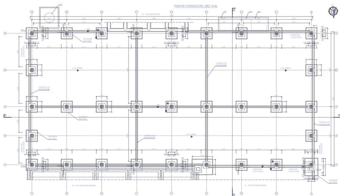
FIGURA 8-19 – PIANTA
