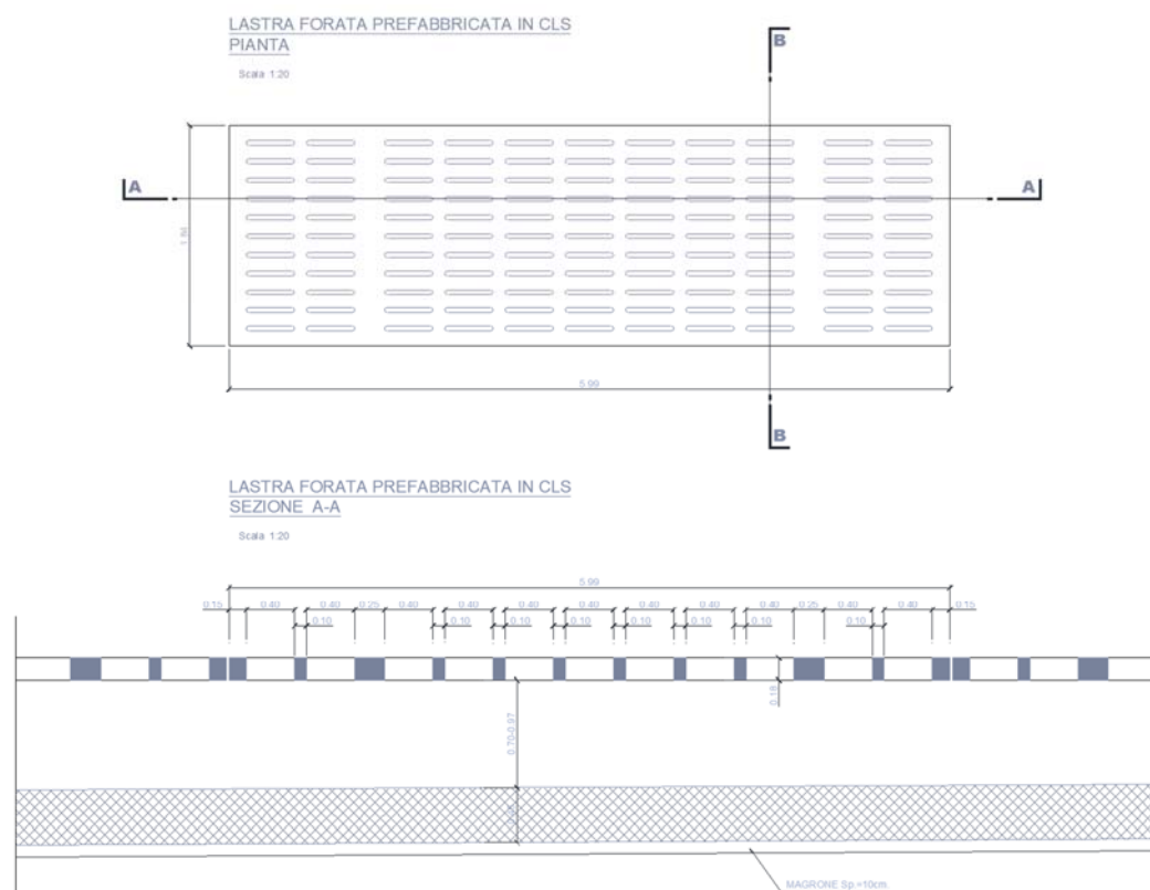
FIGURA 8-10 – LASTRA PREFABBRICATA DI CALPESTIO PER IL BIOFILTRO
