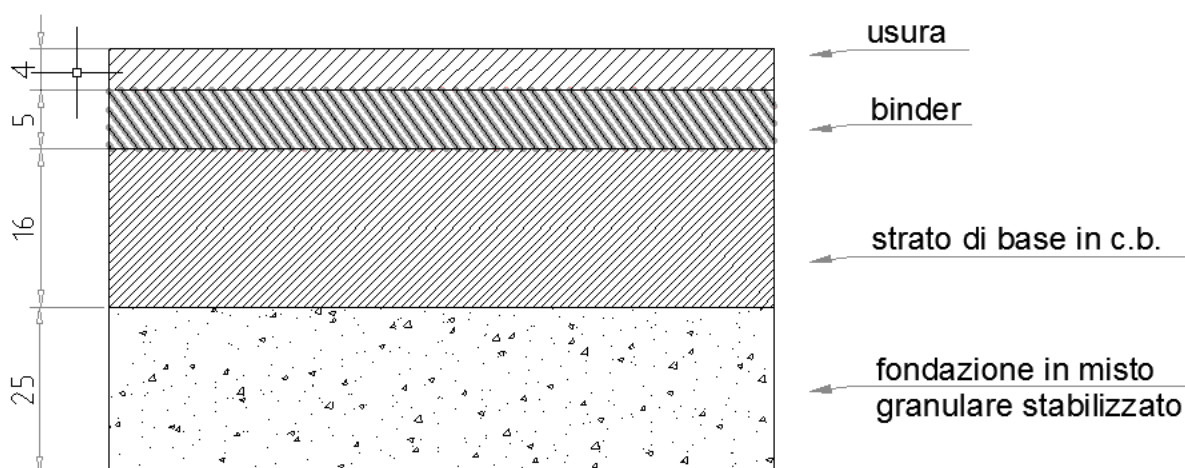
FIGURA 8-41 – SOVRASTRUTTURA
