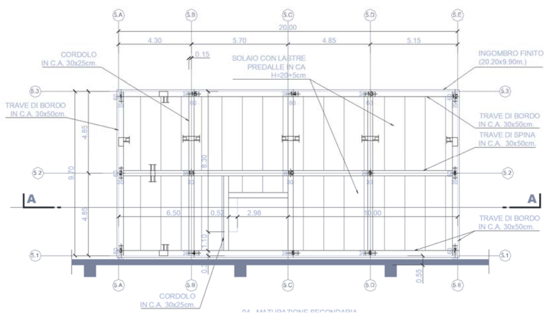
FIGURA 8-26 – PIANTE PRIMO SOLAIO
