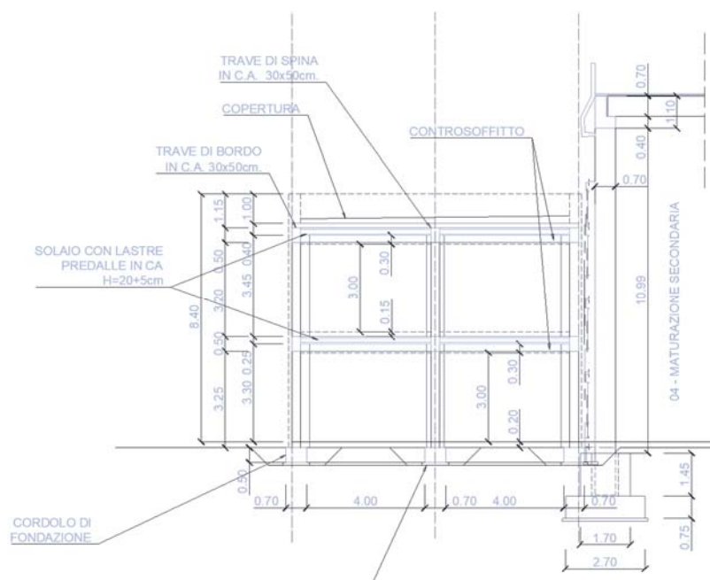
FIGURA 8-29 – SEZIONE TRASVERSALE
