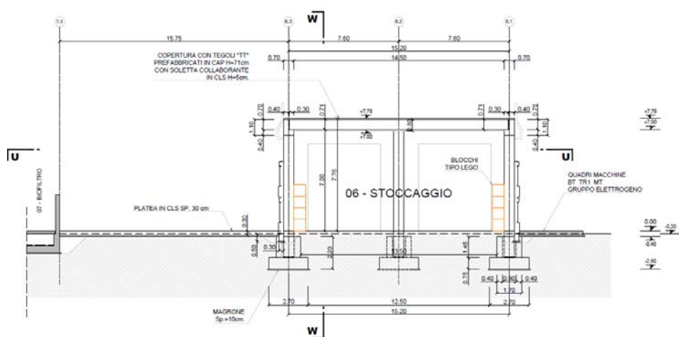
FIGURA 8-22 – SEZIONE TRASVERSALE STOCCAGGIO
