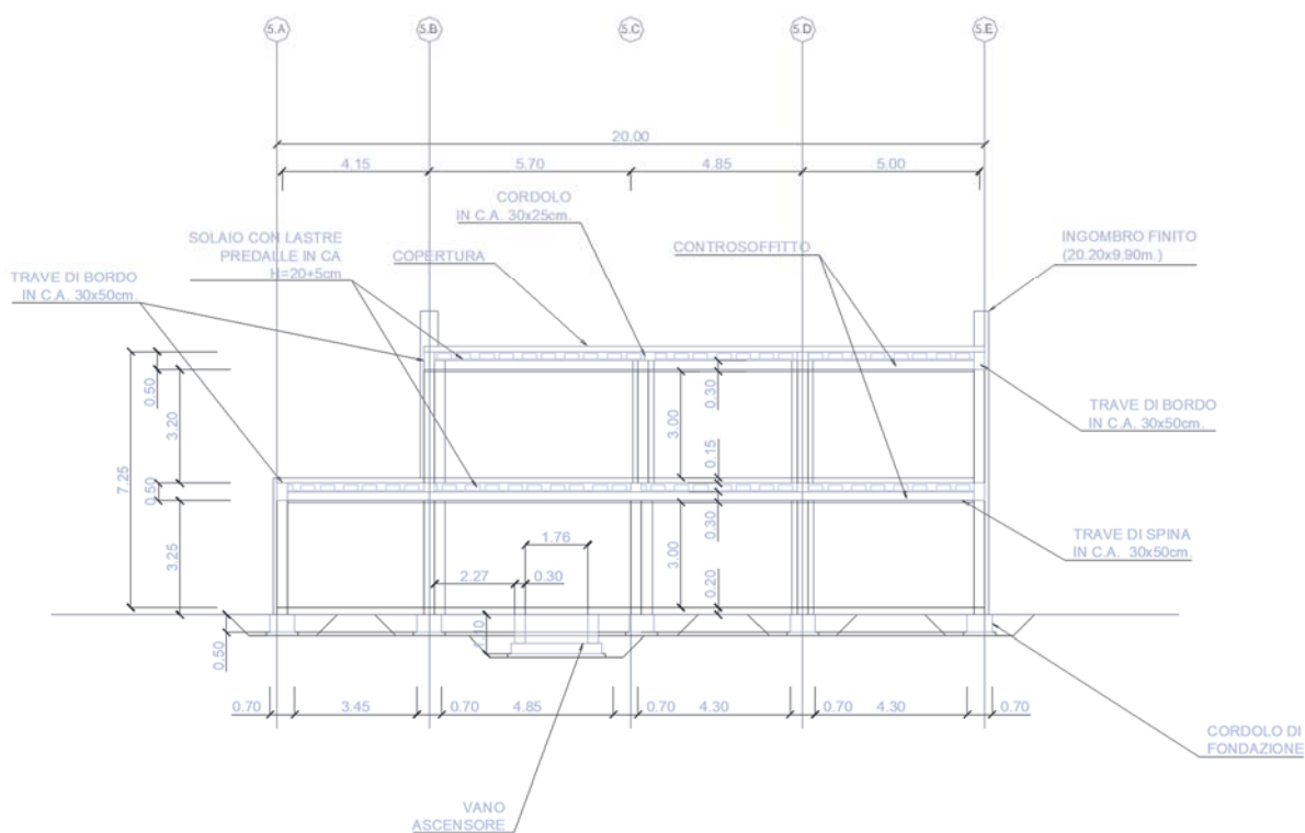
FIGURA 8-28— SEZIONE LONGITUDINALE
