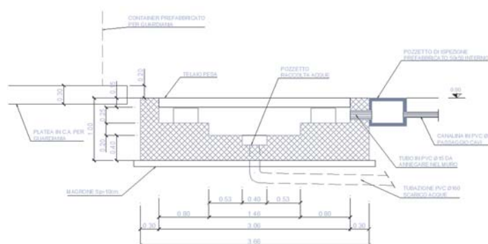
FIGURA 8-31 – SEZIONE TRASVERSALE
