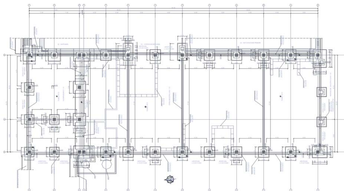
FIGURA 8-14 – PIANTA
