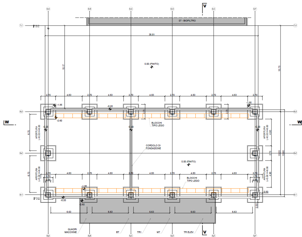
FIGURA 8-21 – PIANTA
