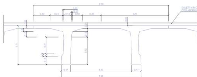
FIGURA 8-3 – SEZIONE TIPO SOLAIO DI COPERTURA
