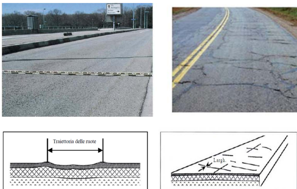
FIGURA 8-40 – ESEMPIO DI DIFETTI DOVUTI A MANCANZA DI PORTANZA: ORMAIE E FESSURAZIONI
