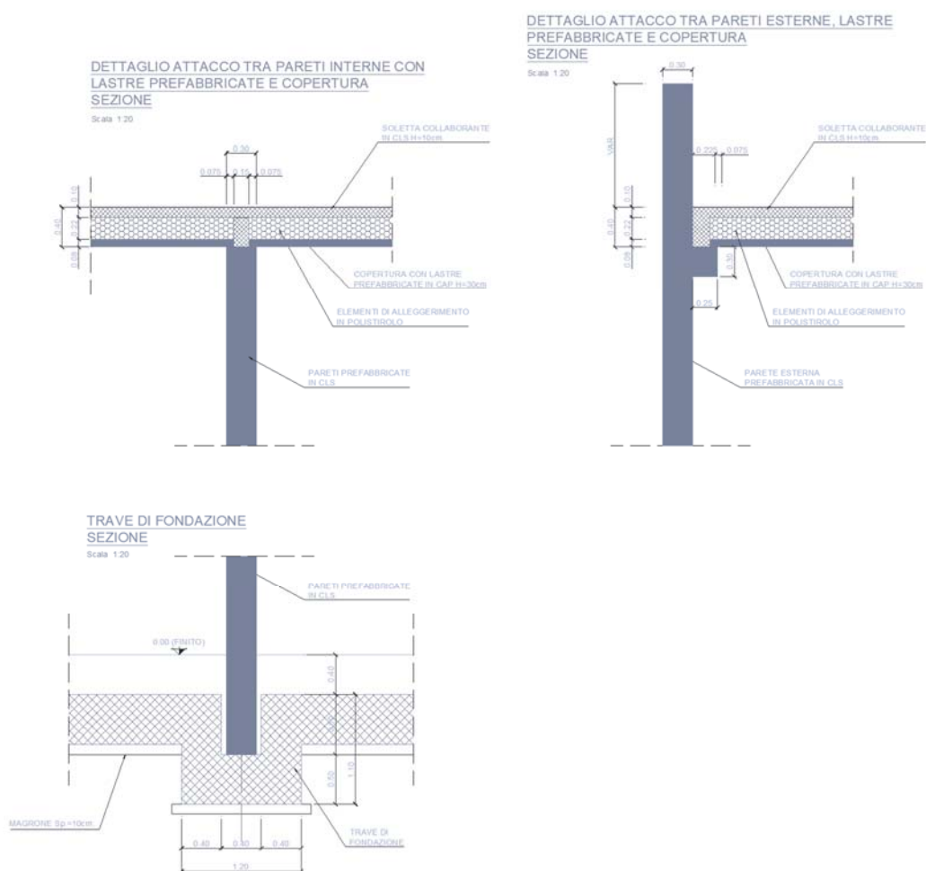
FIGURA 8-17— DETTAGLI TIPICI
