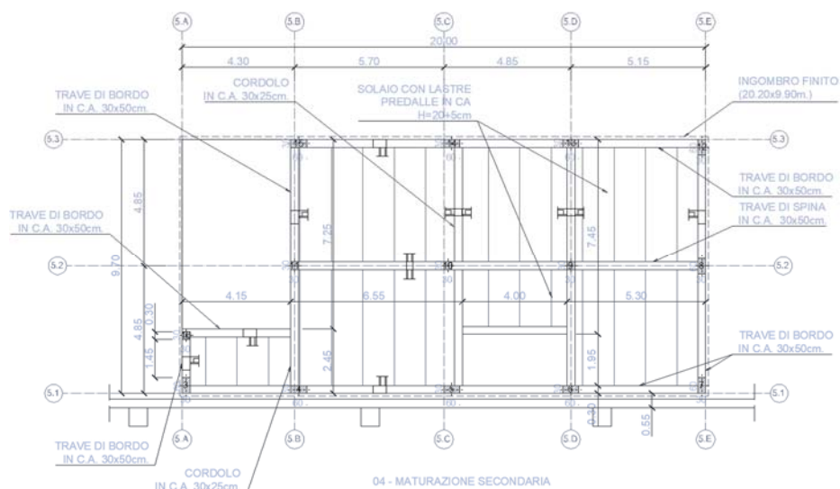
FIGURA 8-27—PIANTA SECONDO SOLAIO
