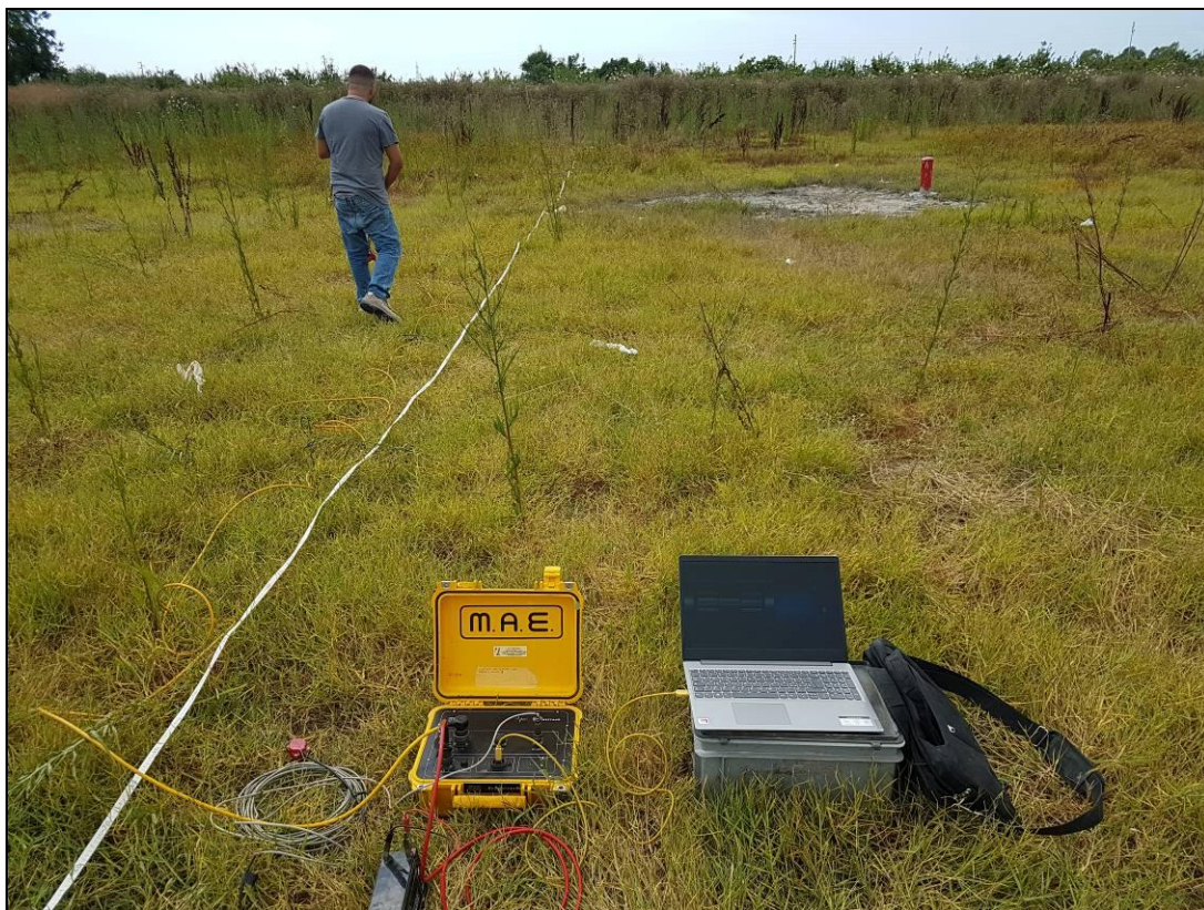
Indagine Sismica MASW
