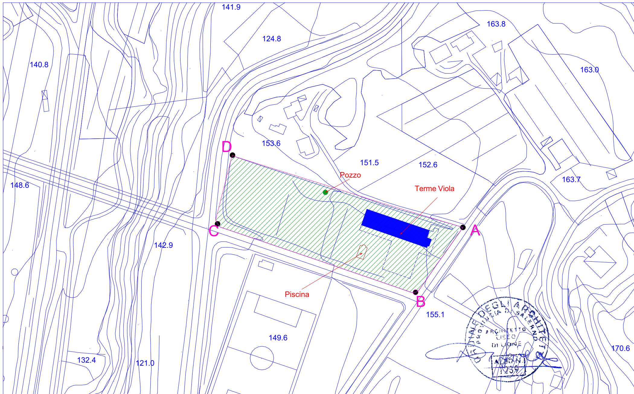
Dettaglio Carta Tecnica Regionale scala 1: 2000
