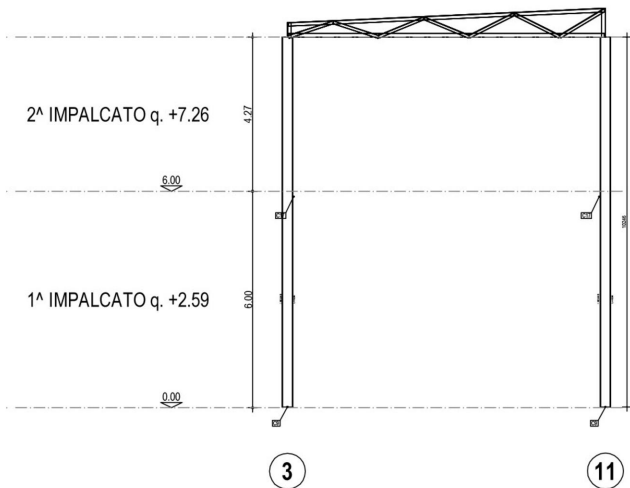
Telaio 3-11
