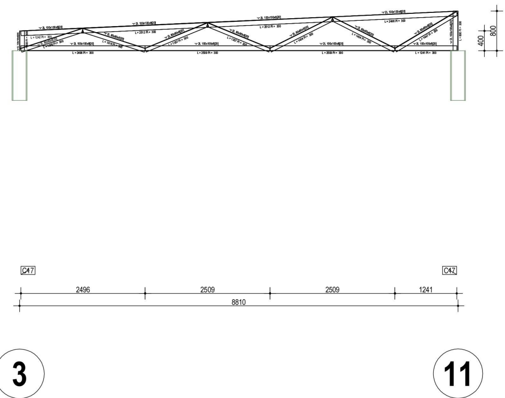
Capriata 1
