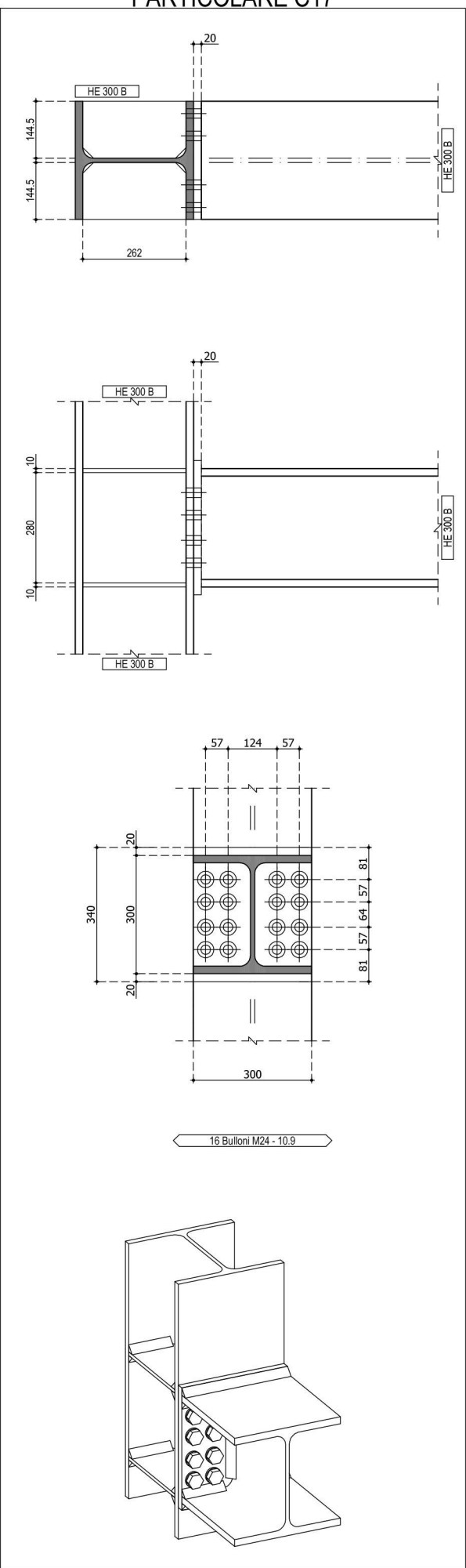
PARTICOLARE C17
