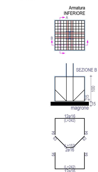
PLINTI 2 Fondazione
