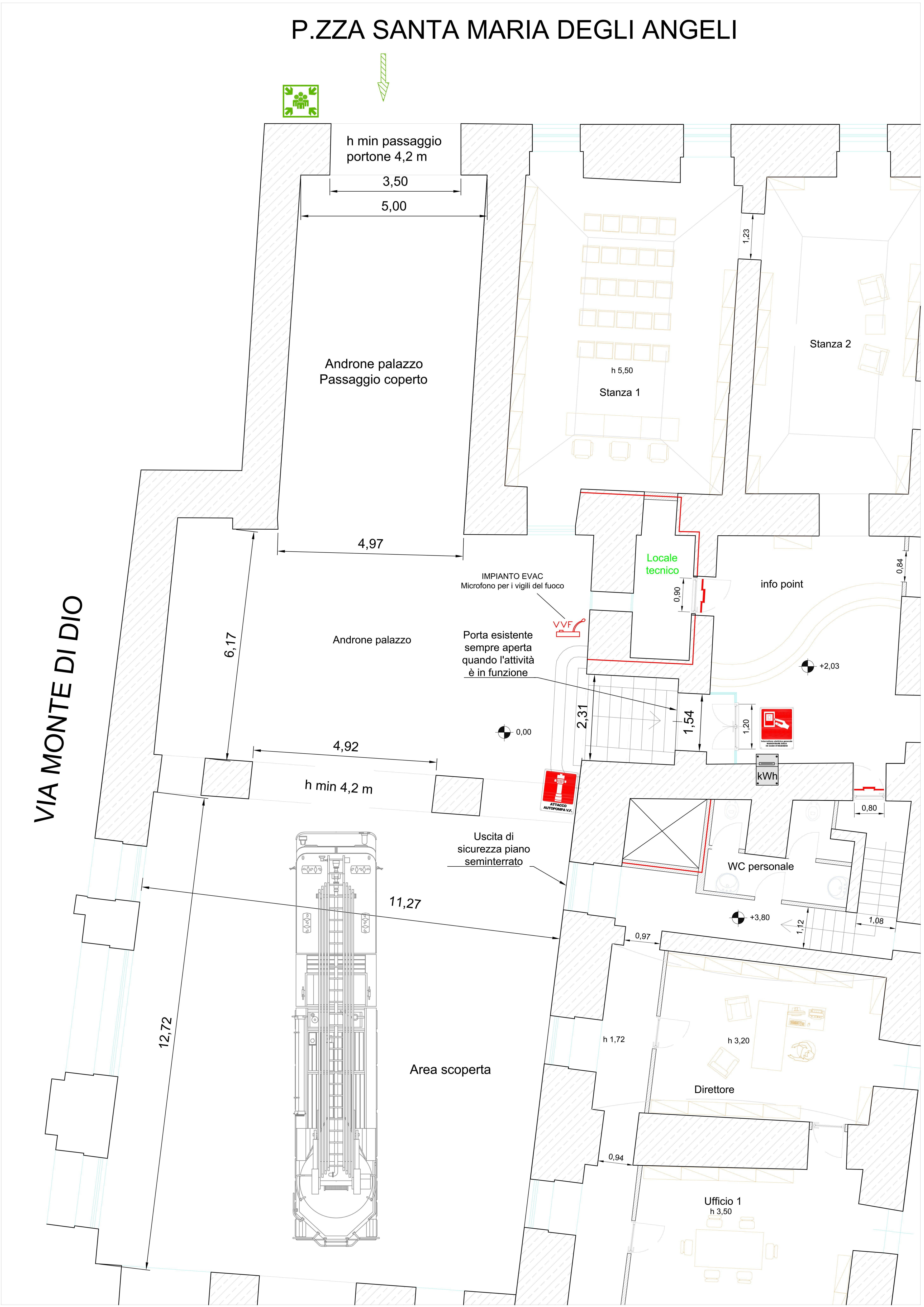
Planimetria Ingresso androne - scala 1:50
