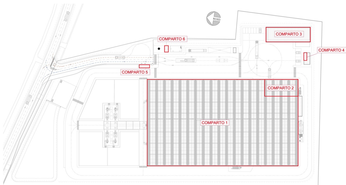
PLANIMETRIA DI RIFERIMENTO COMPARTI INDIVIDUATI
