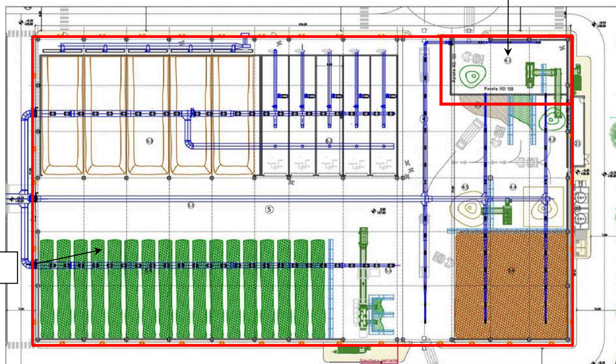
Figura - 13. – Planimetria riferimento attività 70.2.C
