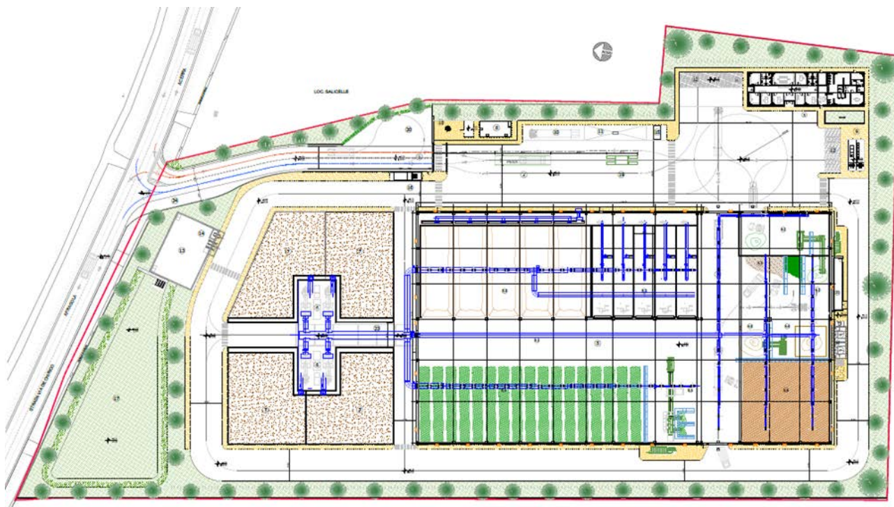
Figura - 6. Layout impianto di progetto
