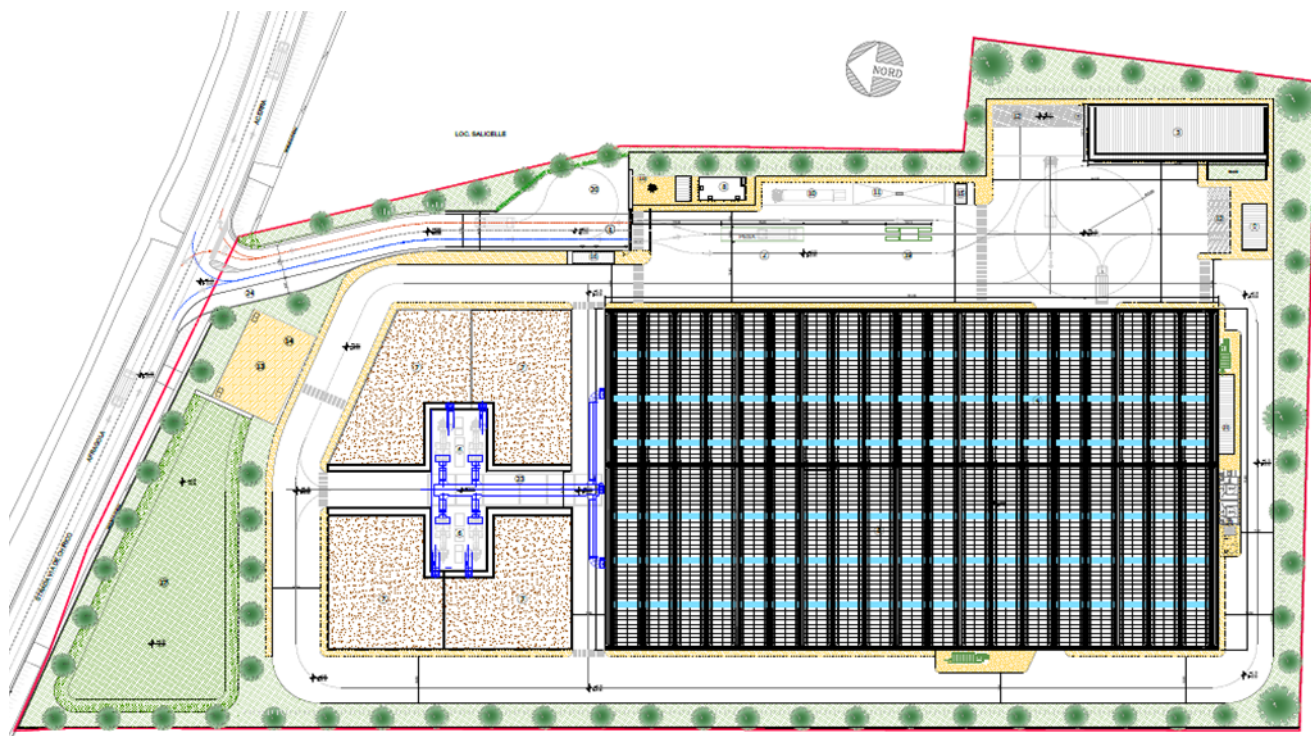
Figura - 5. Planimetria generale dell'impianto
