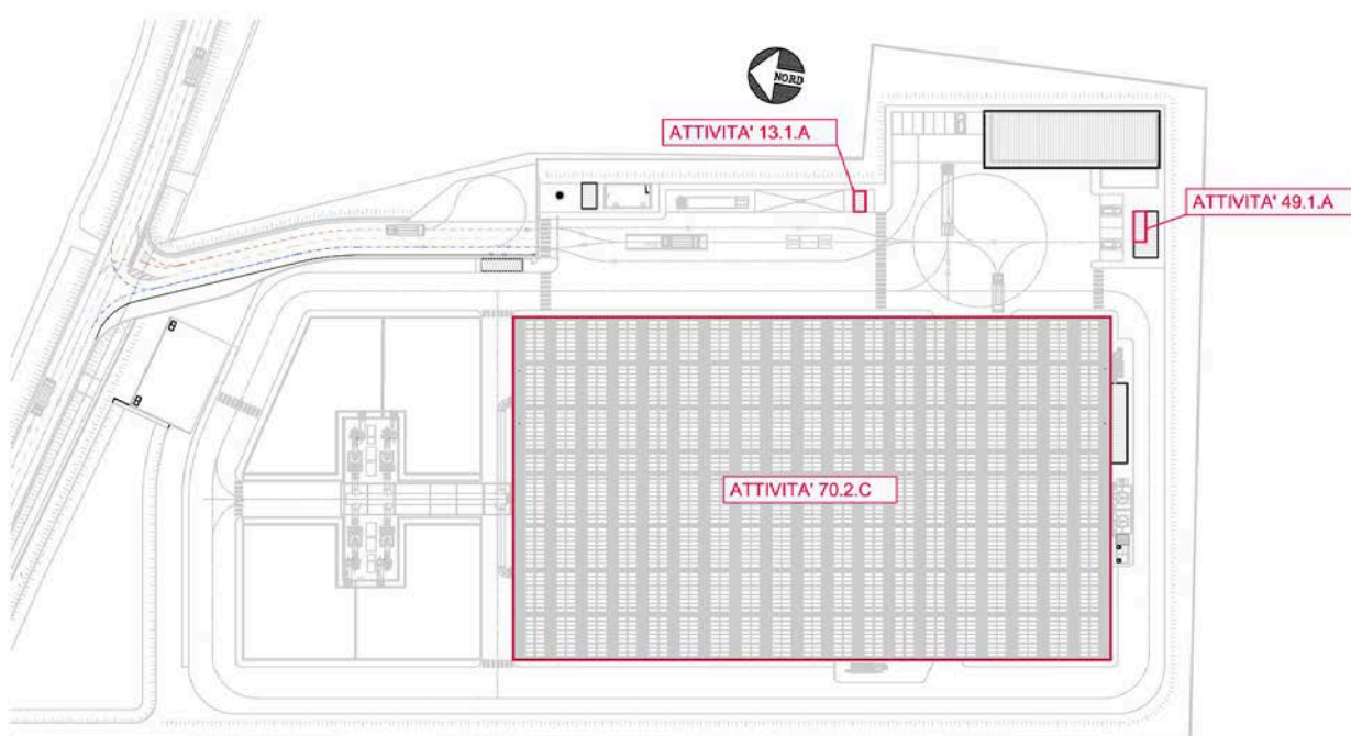
PLANIMETRIA DI RIFERIMENTO ATTIVITA' SOGGETTE PREVENZIONE INCENDI
