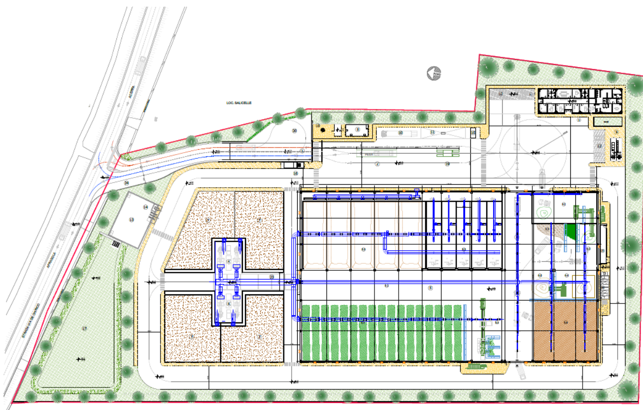
Layout impianto
