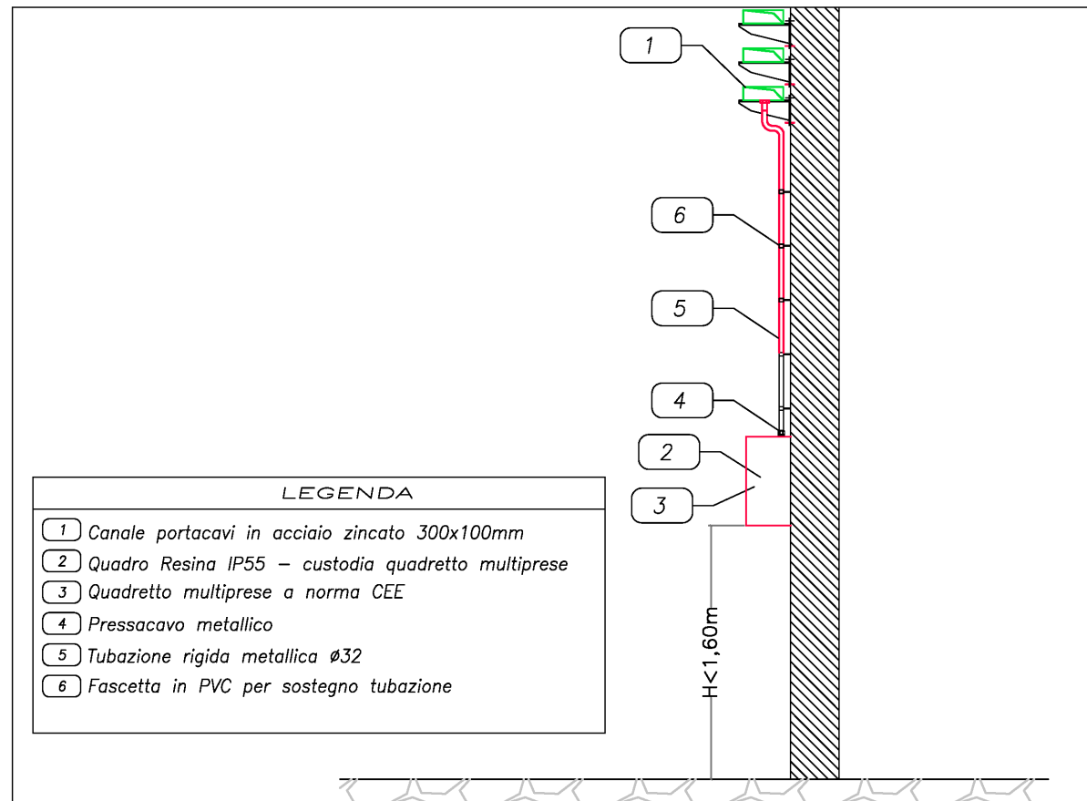
TIPICO ALIMENTAZIONE QUADRO MULTIPRESE
