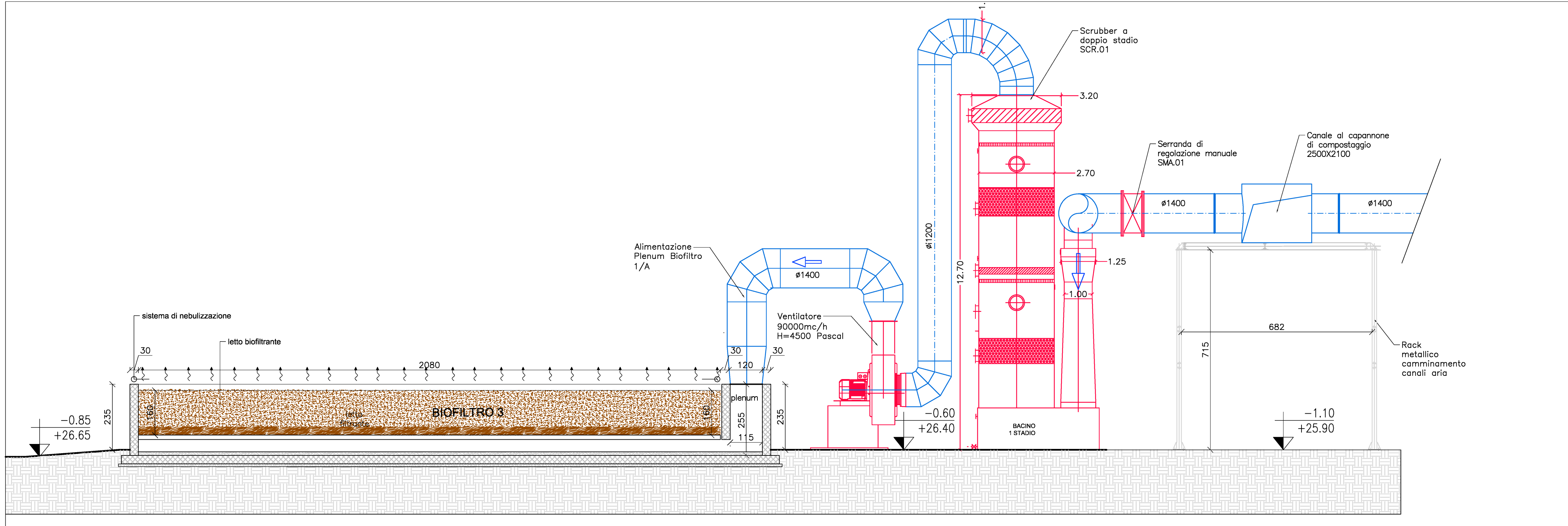
SEZIONE A - A SCRUBBERE N°1/ 2 _ BIOFILTRO 1/2 SCALA 1:100
