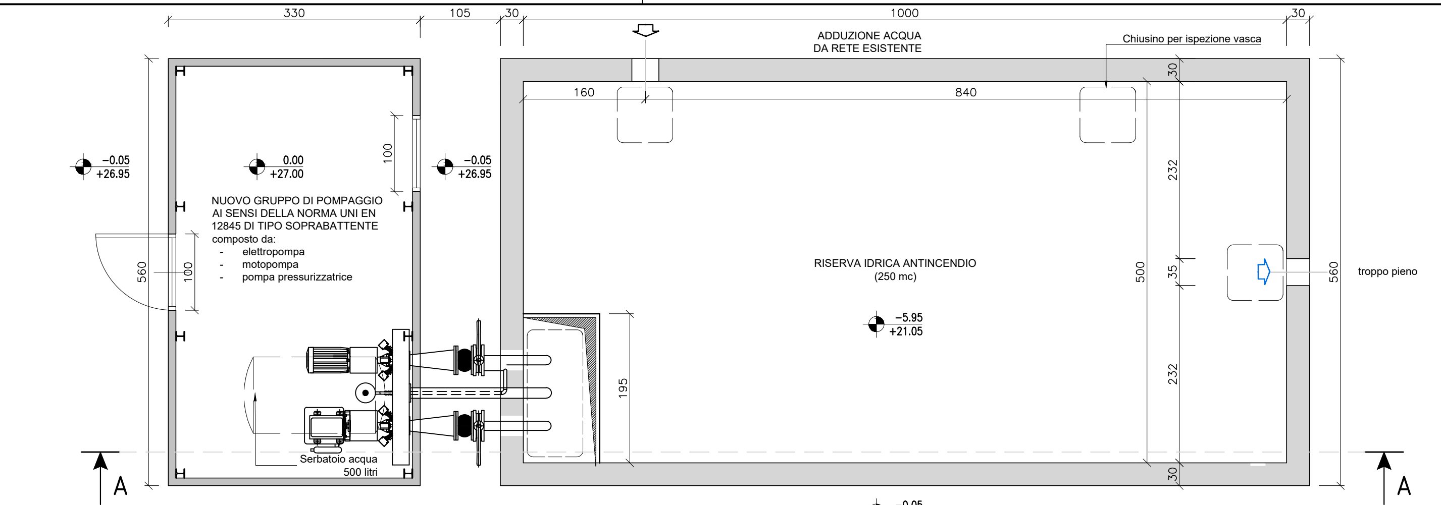
PIANTA SCALA 1:50
