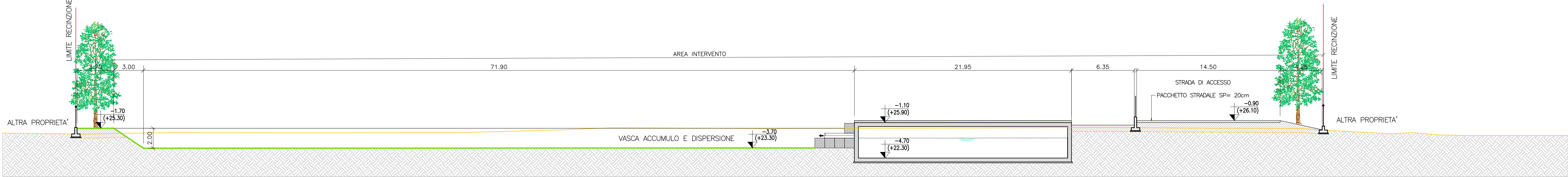
SEZIONE 1-1 SCALA 1:200
