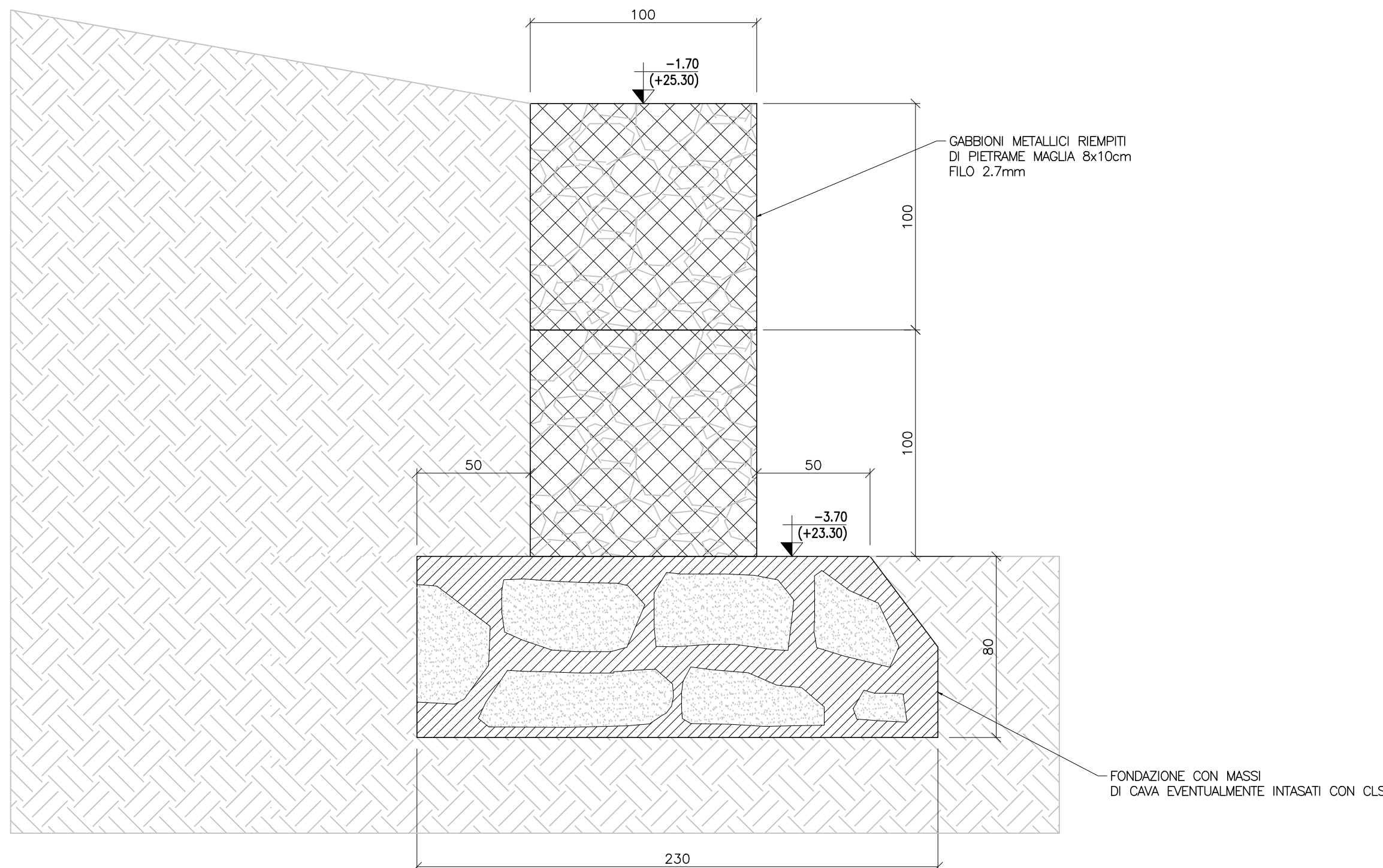
DETTAGLIO GABBIONI - TIPICO SCALA 1:20
