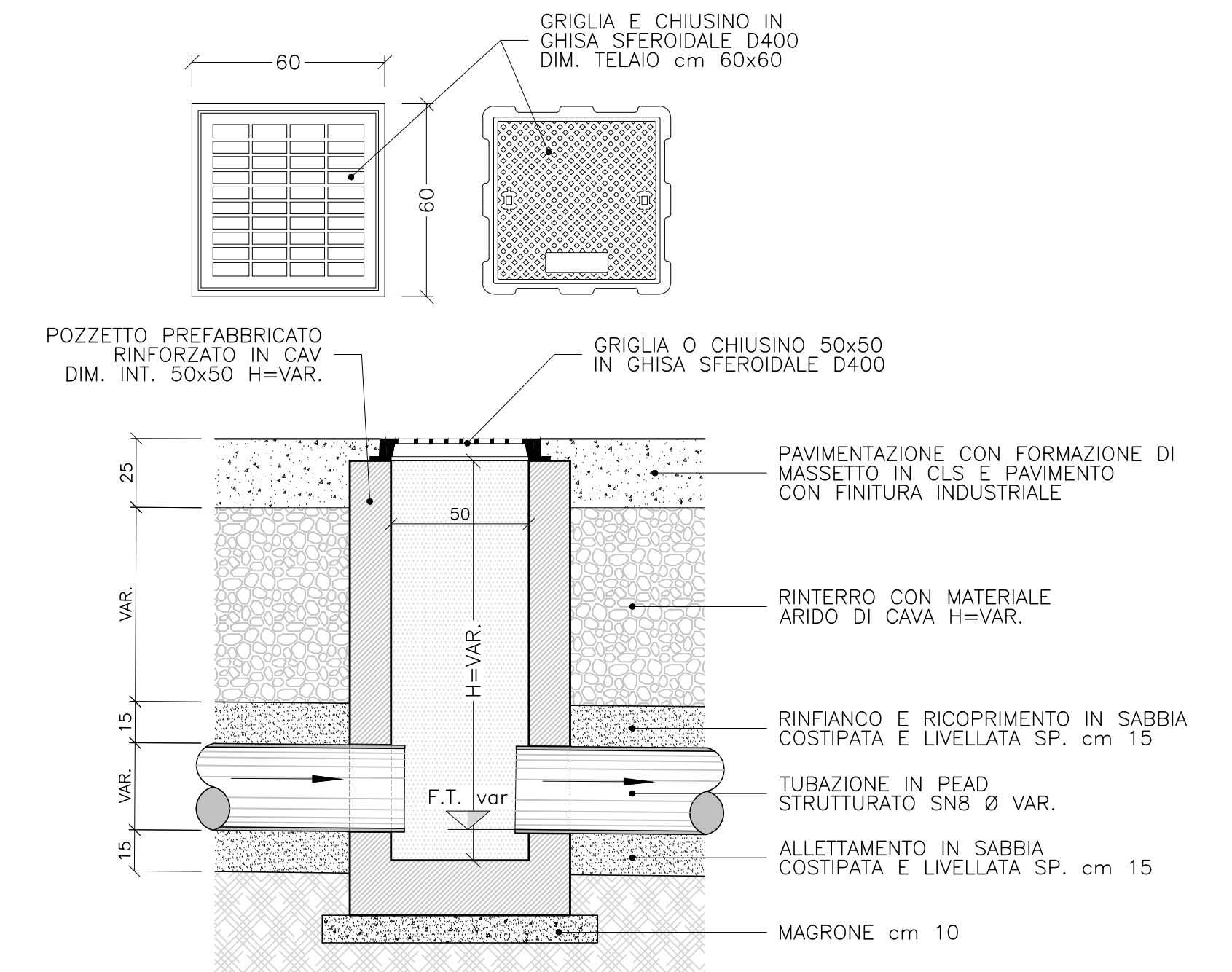
SEZIONE TIPO - POZZETTO 50x50 SCALA 1:20
