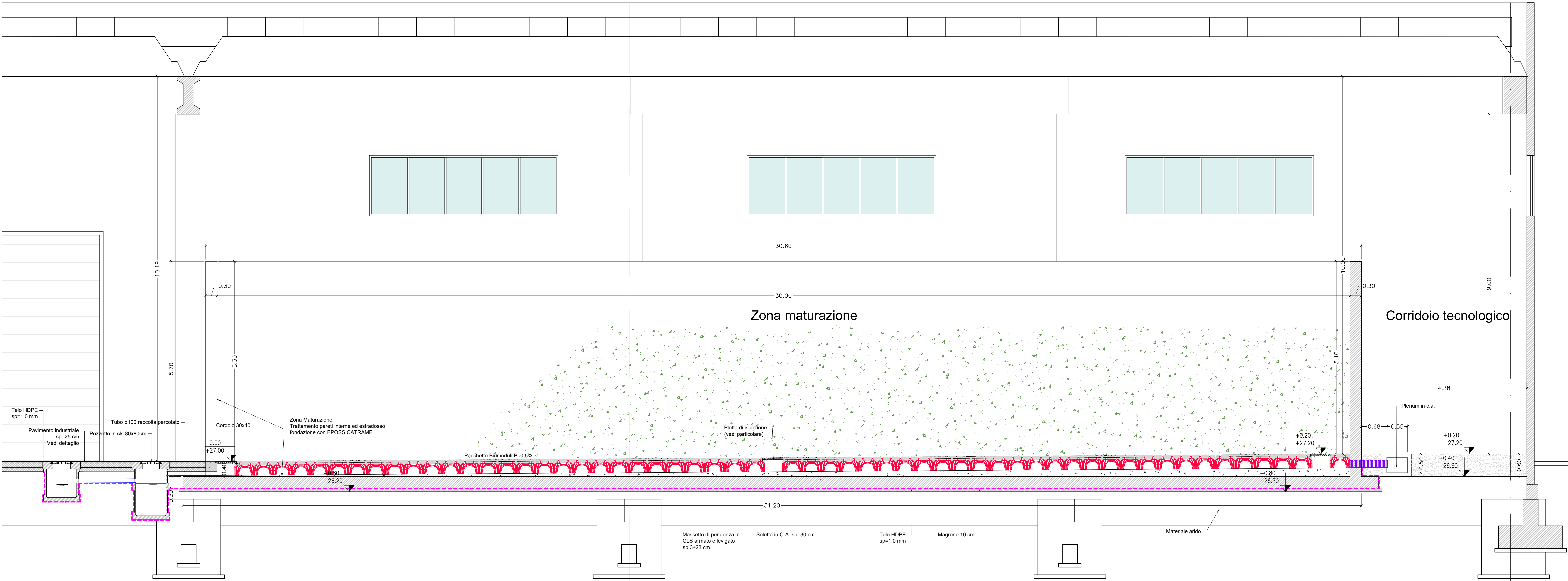
SEZIONE B - B MATURAZIONE PRIMARIA SCALA 1:50
