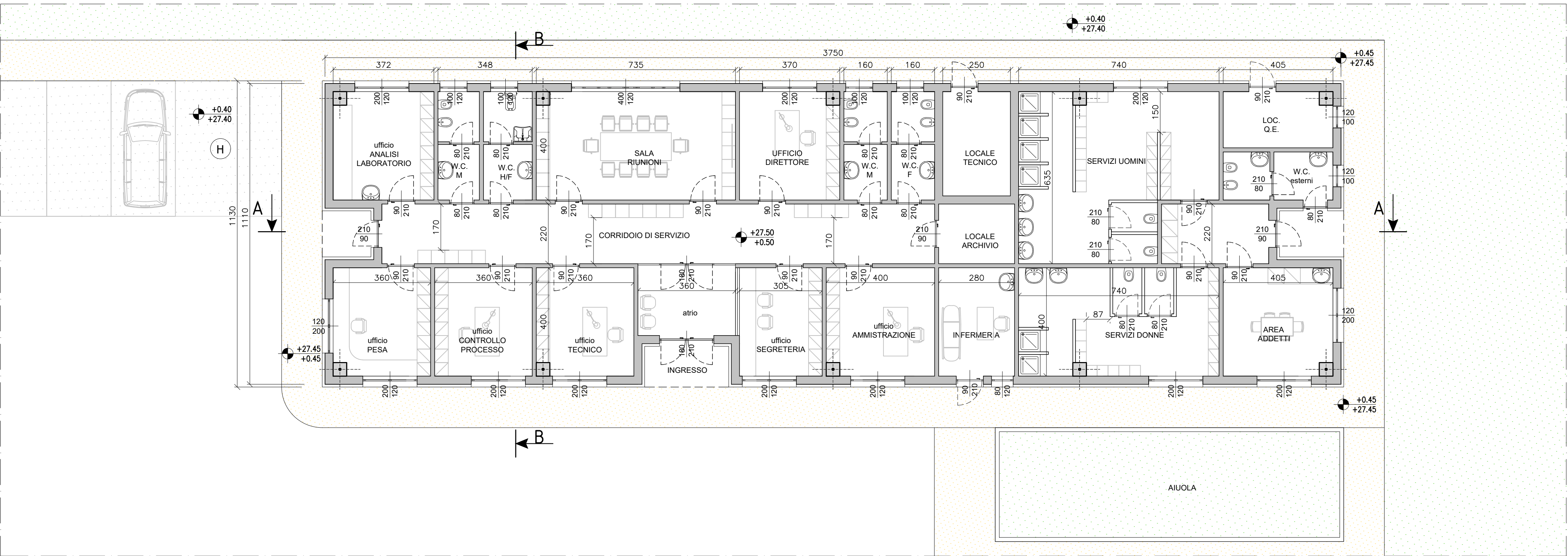
PIANTA PIANO TERRA SCALA 1:100
