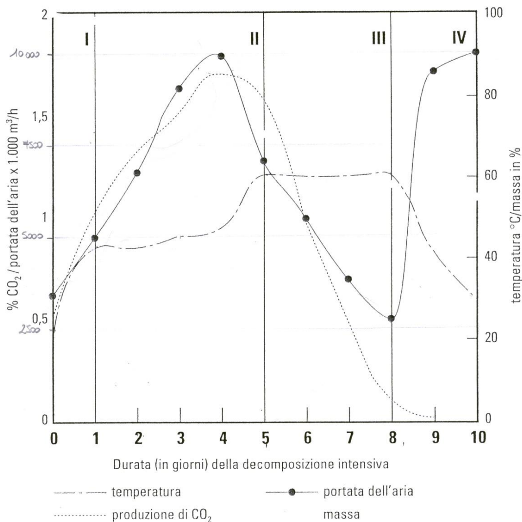
Figura 9 Evoluzione di CO 2 nel processo di compostaggio
