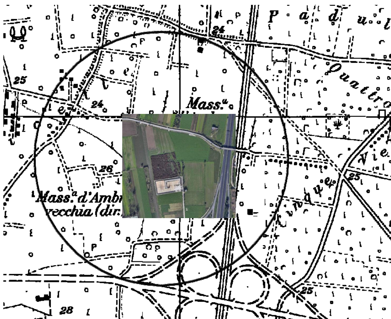
Figura 2 Sovrapposizione stralcio ortofoto con CTR dell'area di intervento
