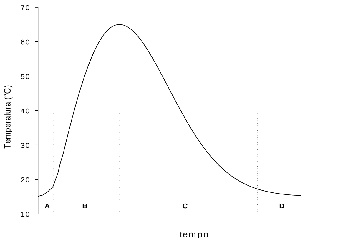
Figura 7 A = Stadio mesofilo; B = Stadio termofilo; C = Stadio di raffreddamento; D = Stadio di maturazione.
