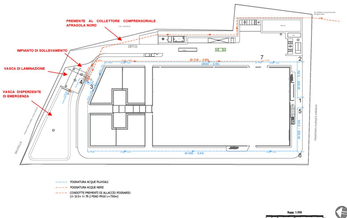
Figura 3 Planimetria rete fognaria
