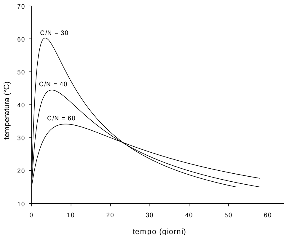
Figura 6 Sviluppo delle reazioni di biodegradazione in funzione del rapporto C/N
