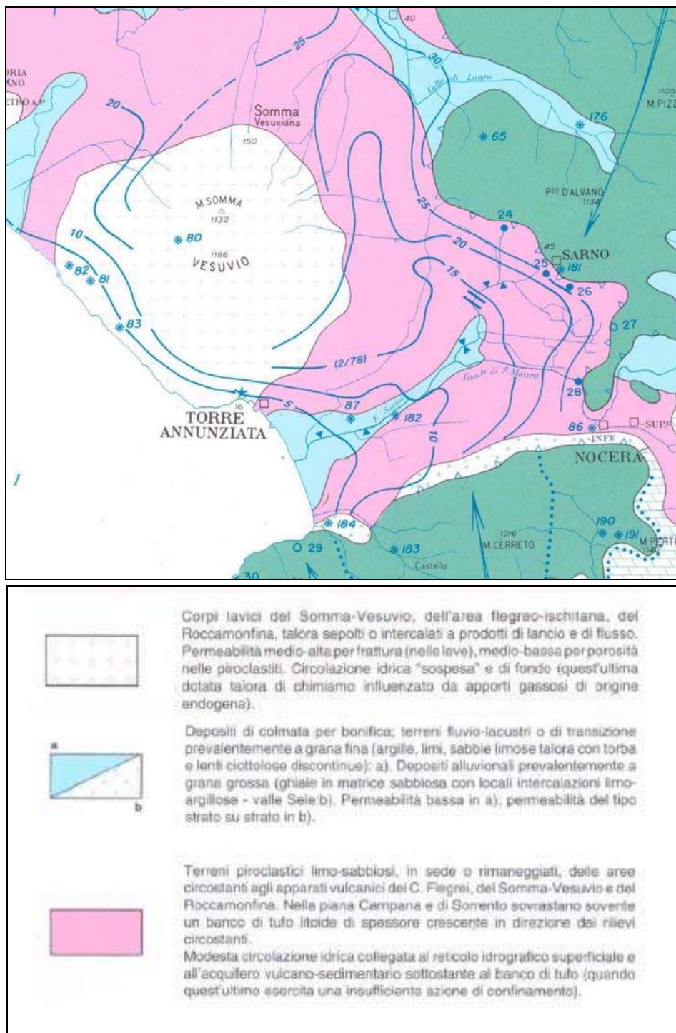
Fig. n. 3 – Complessi litologici
