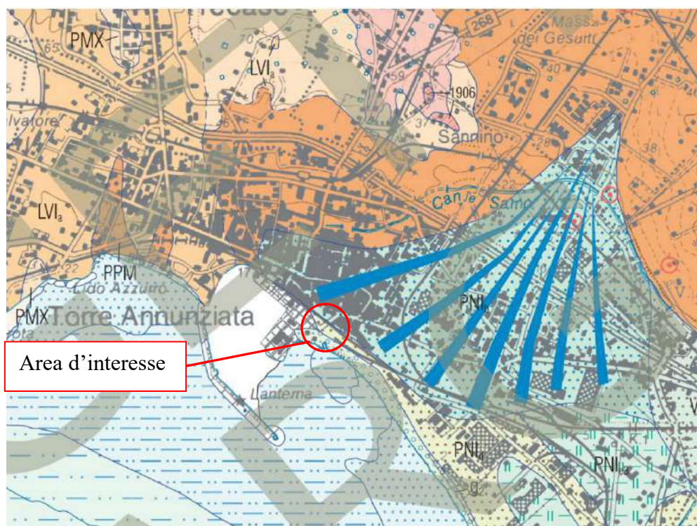
Figura 4 –Stralcio Carta Geologica d'Italia, F. 466 - Sorrento
