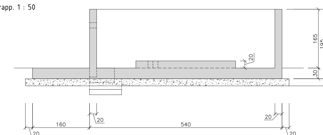
Sezione A-A rapp. 1 : 50
