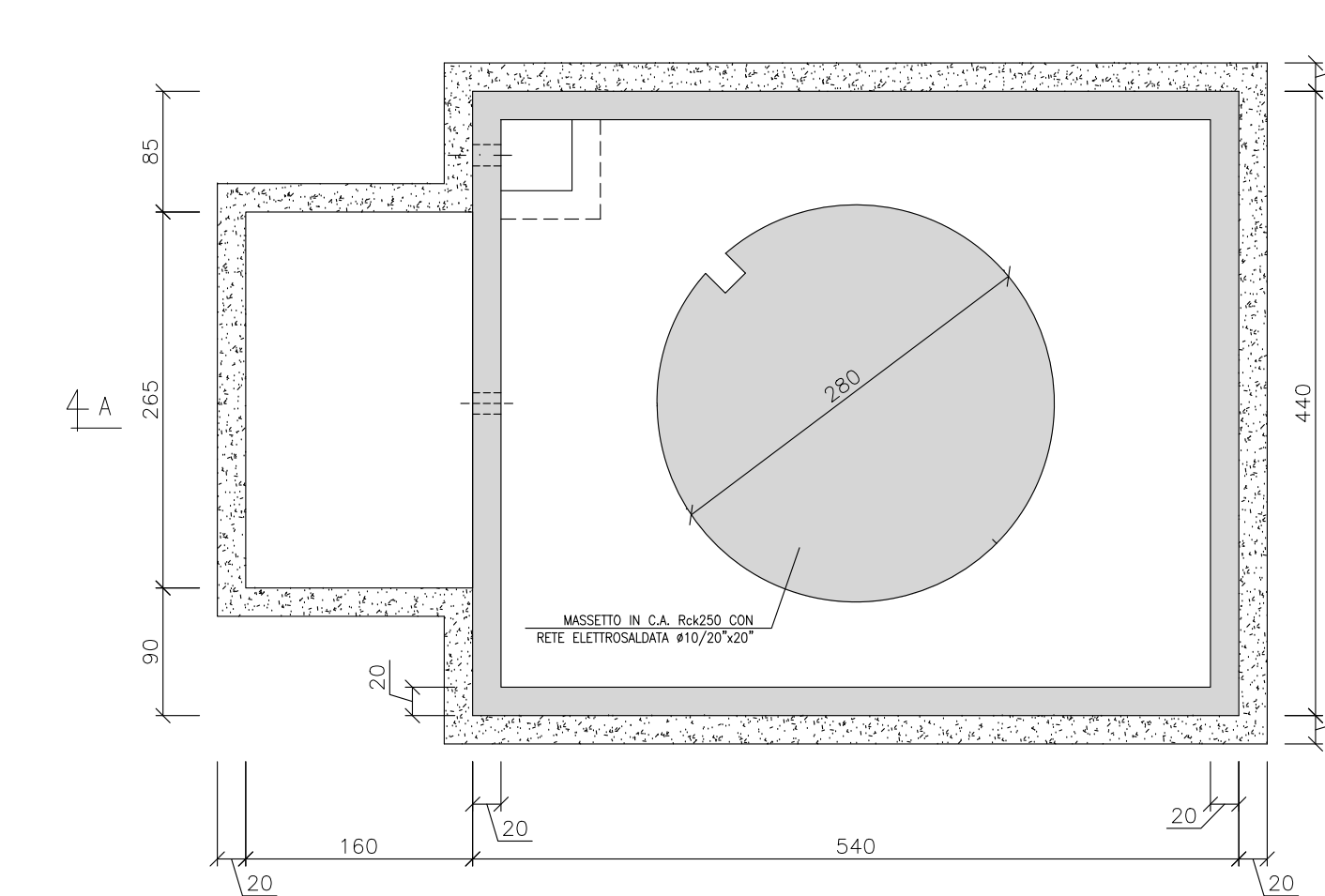
Pianta rapp. 1 : 50
