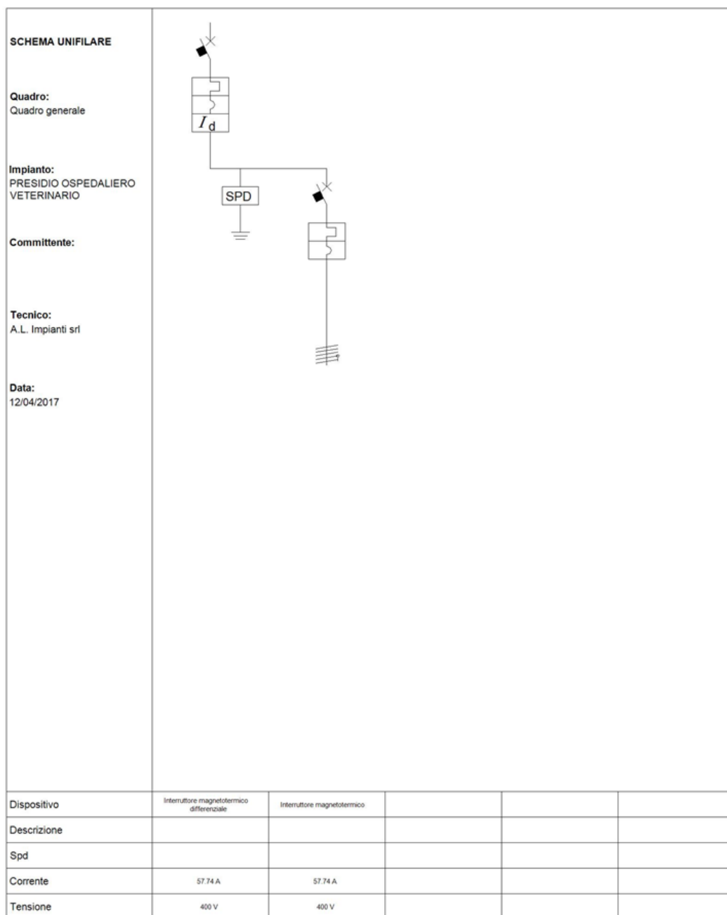
Fig. 5: Schema unifilare quadro "Quadro generale"
