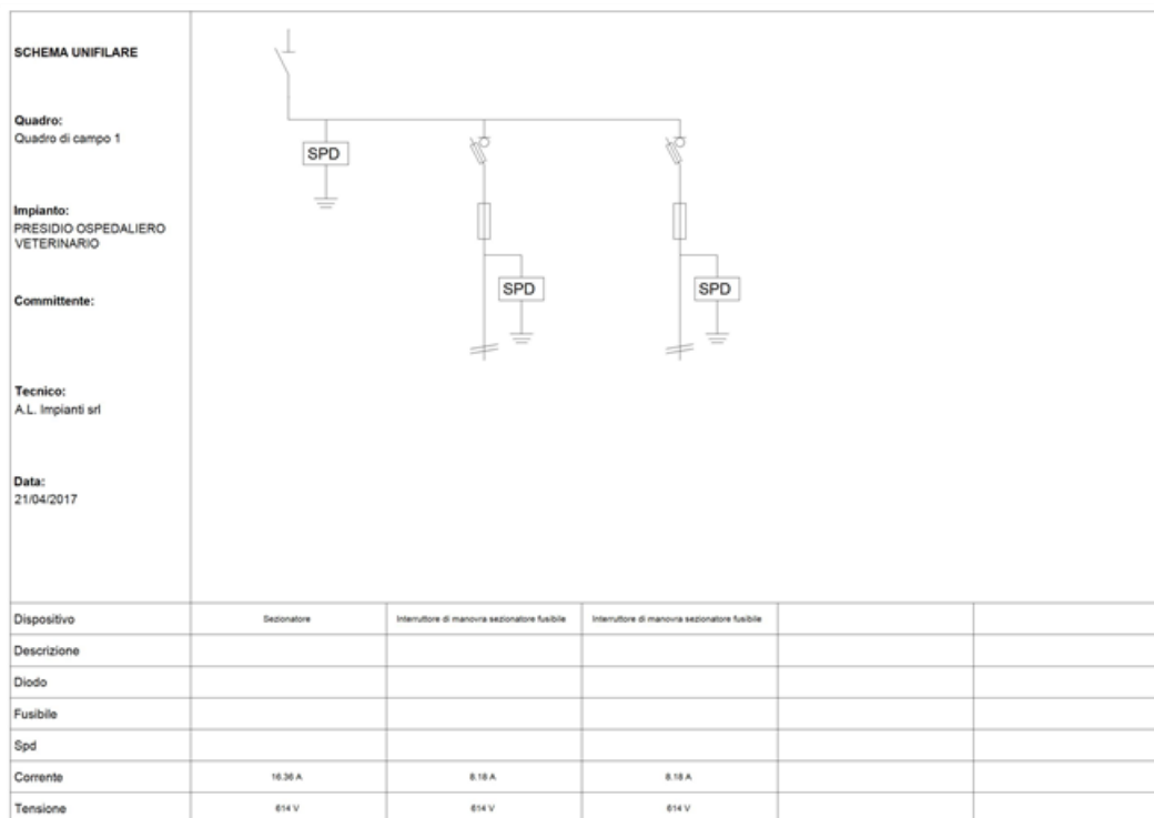
Fig. 7: Schema unifilare quadro "Quadro di campo 1"
