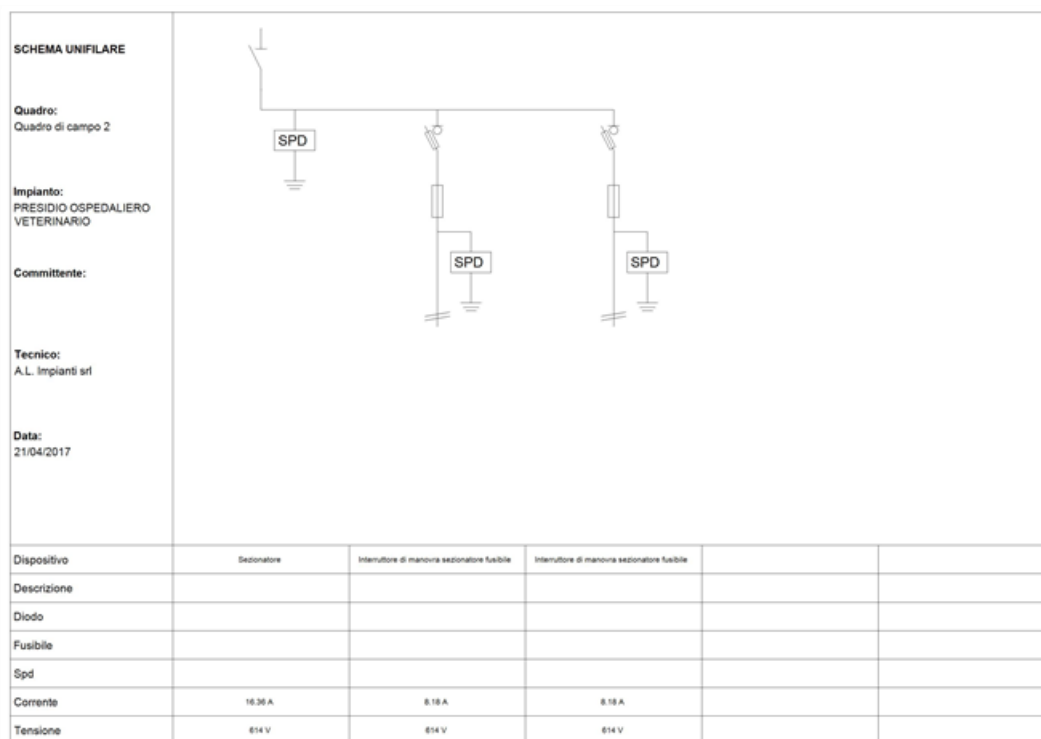
Fig. 8: Schema unifilare quadro "Quadro di campo 2"
