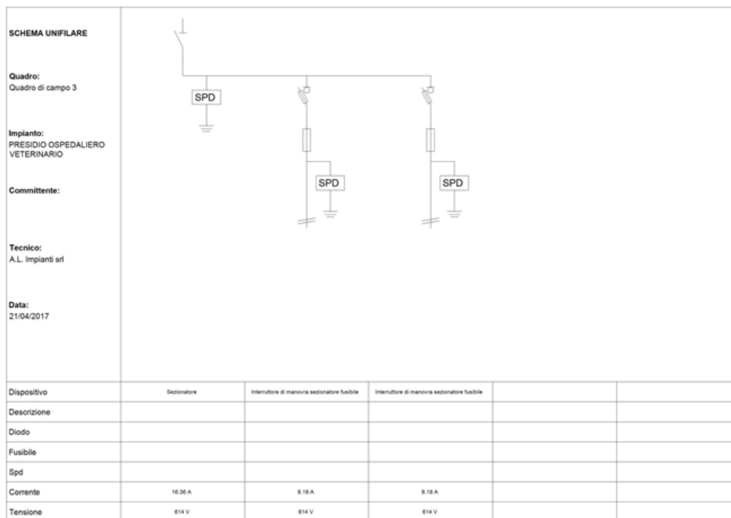
Fig. 9: Schema unifilare quadro "Quadro di campo 3"
