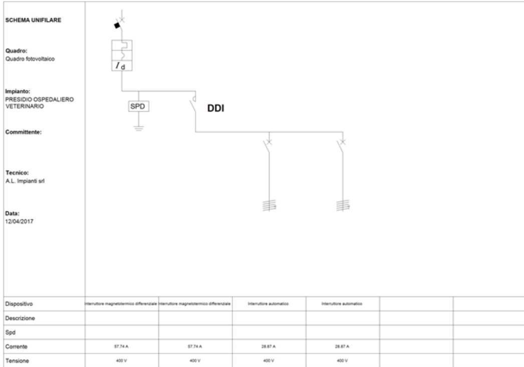
Fig. 6: Schema unifilare quadro "Quadro fotovoltaico"
