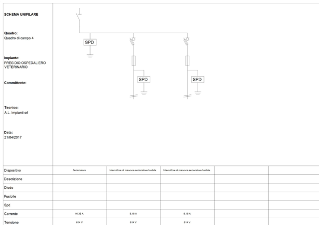
Fig. 10: Schema unifilare quadro "Quadro di campo 4"
